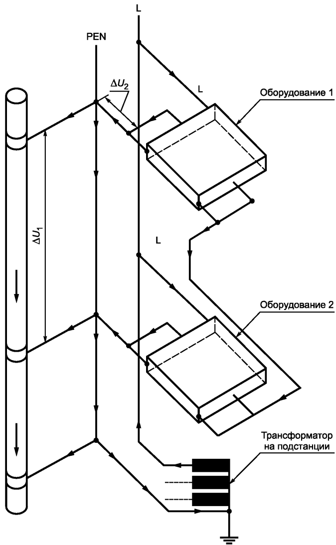
Рисунок 2а — Система заземления типа TN-C
