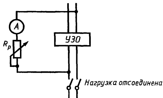
Рисунок В.2 — Схема проверки УЗО по методу 2
