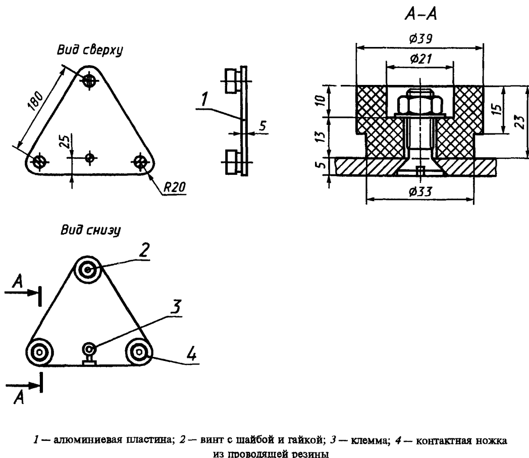
Рисунок А.1 — Испытательный электрод 2
