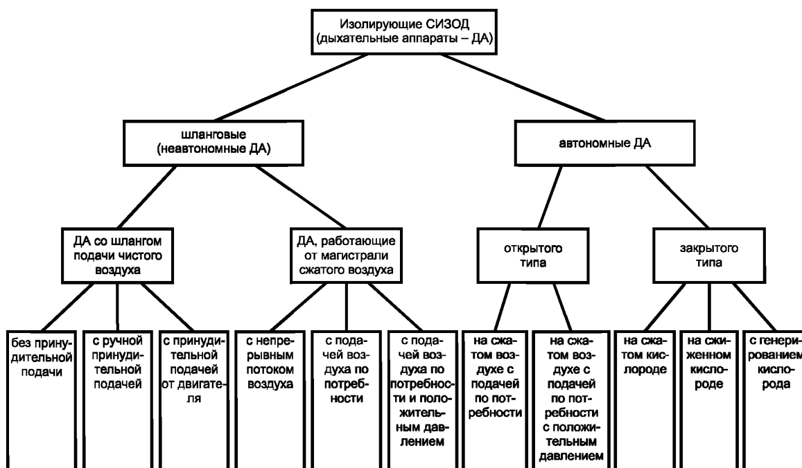
Рисунок 4 — Классификация изолирующих средств индивидуальной защиты органов дыхания
