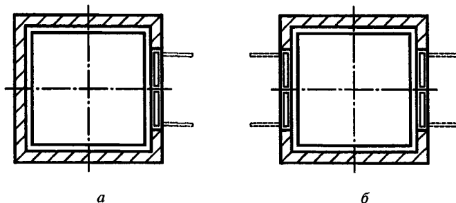
Рисунок 3 — Подъемные платформы
