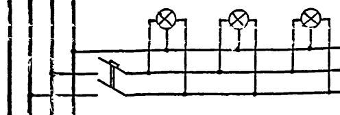
Рис.2. Схемы групповых линий при с/с теме 380/220 и 220/127 В и питании ОП напряжением 380 и 220 В.
