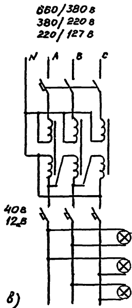
Рис. 4 Схемы сети малого напряжения
