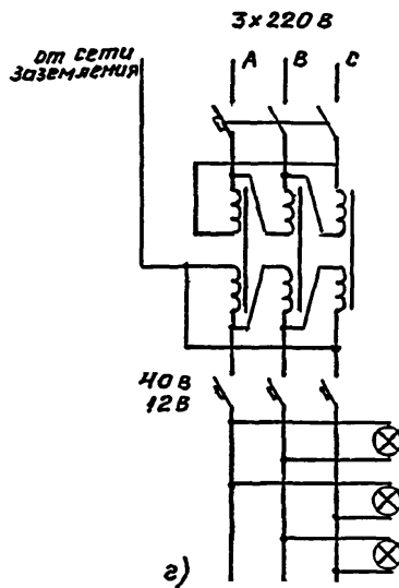
Рис. 4 Схемы сети малого напряжения
