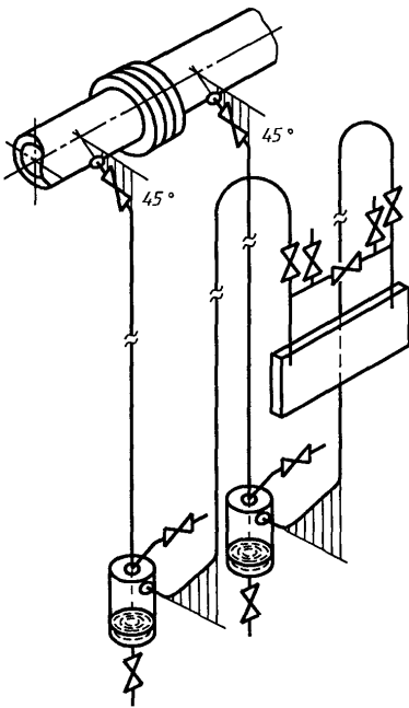
Рисунок В.10 — Дифманометр под трубопроводом (вариант)
