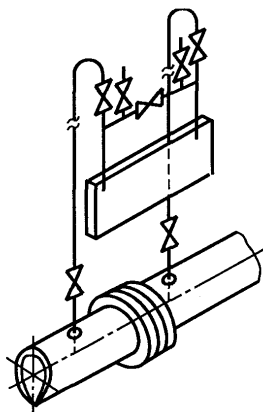
Рисунок В.1 — Дифманометр над трубопроводом
