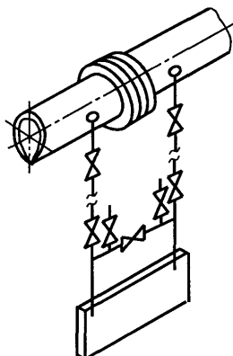
Рисунок В.2 — Дифманометр под трубопроводом
