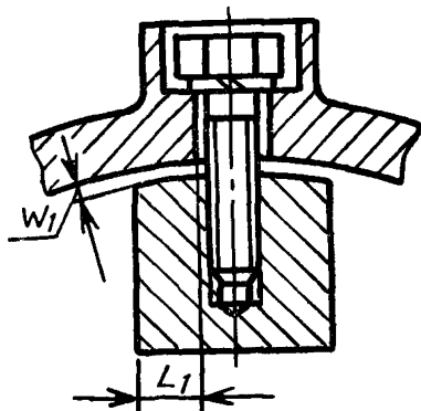
Вариант крепления полюсов электрических машин
