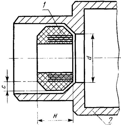
1 — уплотнительное кольцо для кабеля; 2 — корпус кабельного ввода; d — диаметр проходного отверстия; H — высота уплот- нительного кольца; s — толщина уплотни- тельного кольца
