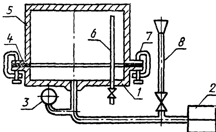
Принципиальная схема для проведения гидравлических испытаний
