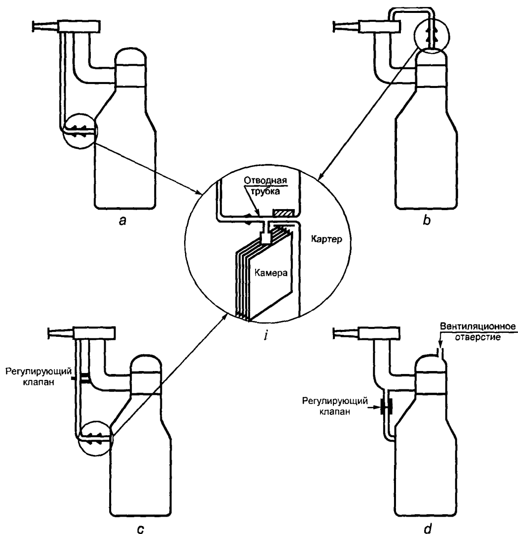
a — прямая рециркуляция при слабом разрежении; в — непрямая рециркуляция при слабом разрежении; с — прямая двухканальная рециркуляция; д — вентиляция картера с применением рециркулирующего клапана (камера должна быть присоединена к вентиляционному отверстию); и — соединение отводной трубки и камеры
