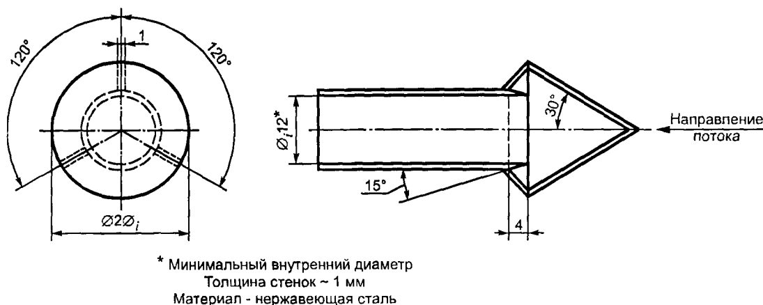
Рисунок 5/2 — Схема пробоотборника твердых частиц
