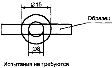
Рисунок 26 — Схема испытания по 24.1.1
