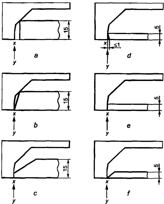
Случаи а) и б) — не соответствуют; случаи с), d), е) и f) — соответствуют (соот- ветствие должно быть проверено требовани- ми 20.8, используя калибр, представленный на рисунке 23)
