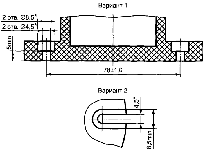
Рисунок С.3 — Выключатель для скрытой установки
