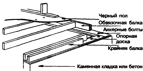
Рисунок 6-4 — Опирающие прогоны (балки) перекрытия на опорную доску, уложенную на фундаментную стену
