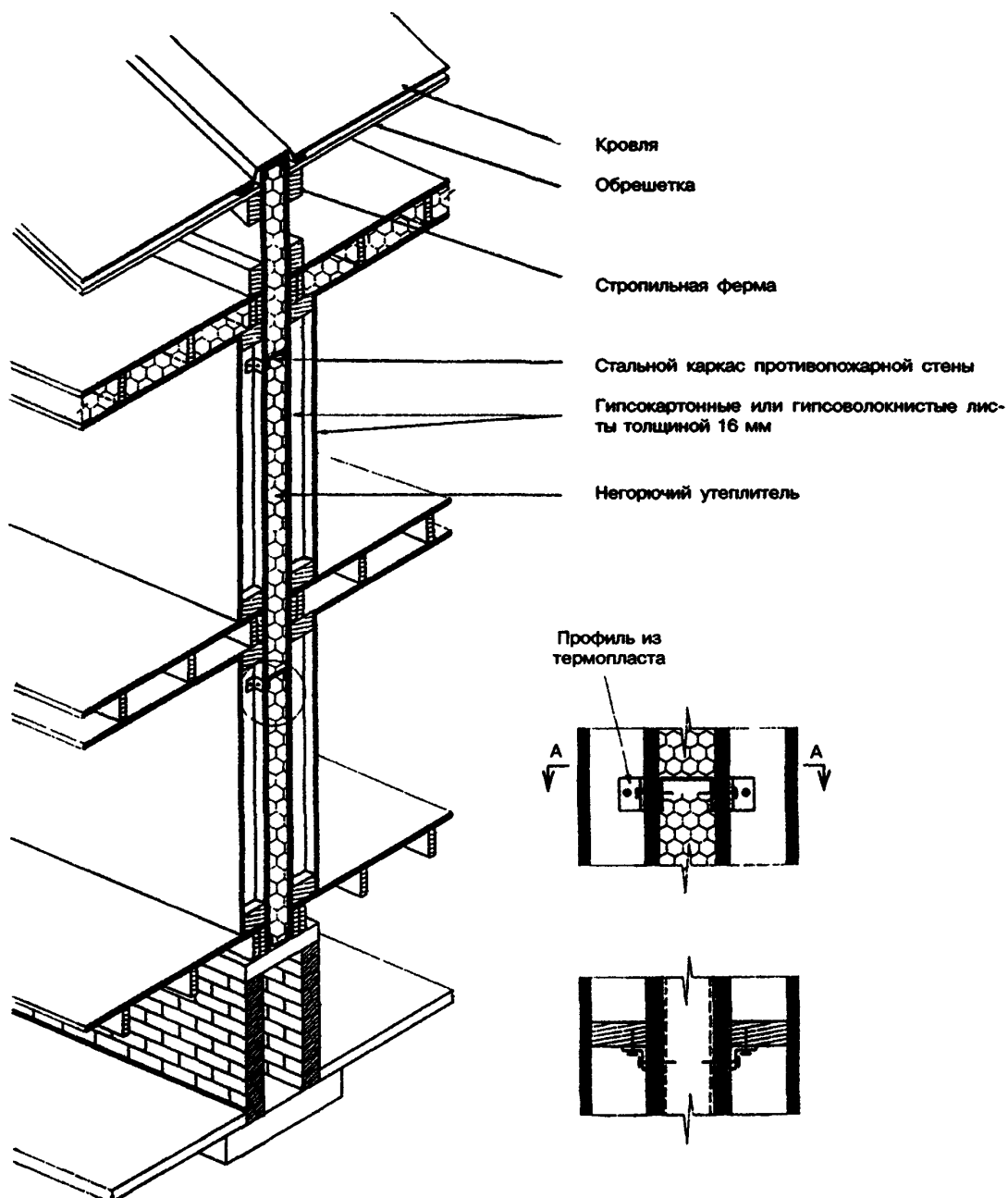
Рисунок 7-6 — Межквартирная противопожарная стена 2-го типа каркасной конструкции
