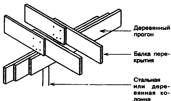
Рисунок 6-7 — Опираие балок перекрытия на деревянный прогон
