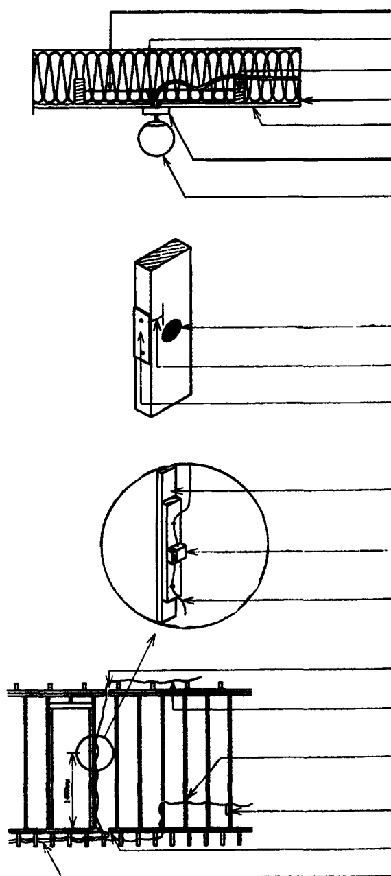
Рисунок 13-9 — Прокладка электрических проводов в элементах каркаса
