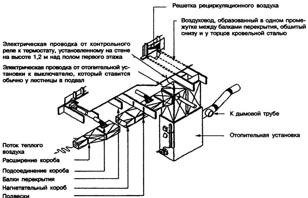
Рисунок 13-4 — Крепление воздуховодов
