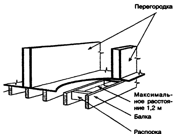
Рисунок 6-13 — Опираание перегородок
