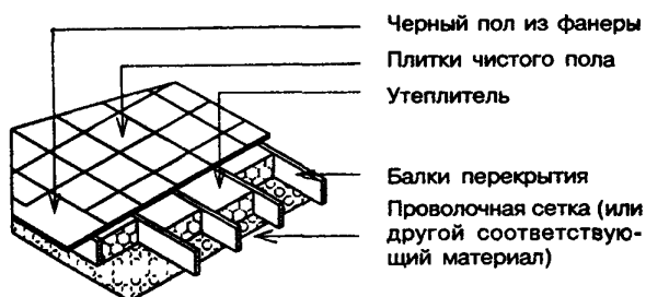
Перекрытие над неотапливаемым подпольем, утепленное насыпным утеплителем
