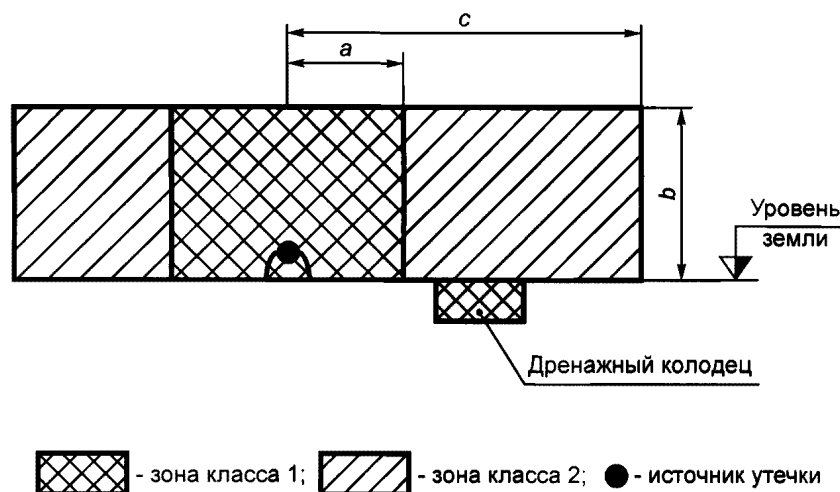
Пример № 2 Насос для перекачки горючей жидкости, установленный снаружи на уровне земли
