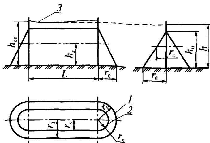
Рис. 11 (к п. 7.4.1). Схема зоны защиты одиночного тросового молниеотвода:
