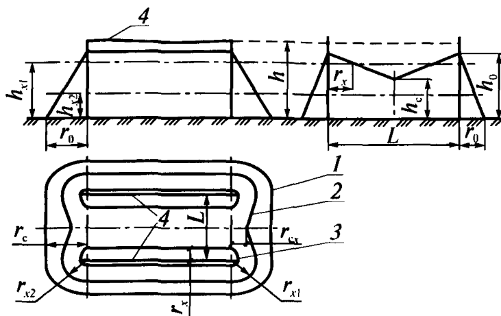
Рис. 12 (к п. 7.5.1). Схема зоны защиты двойного тросового молниеотвода:
