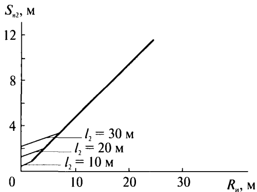
Рис. 5 (к п. 6.3). Наименьшие допустимые расстояния от молниевотвода до защищаемого сооружения
