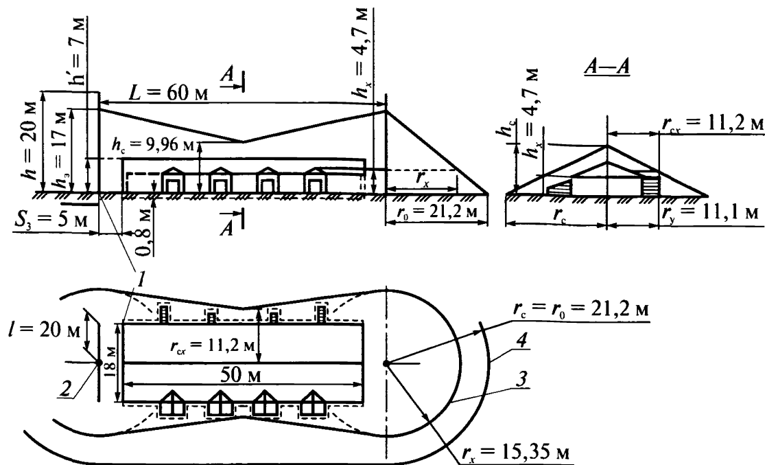
Рис. 18 (к п. 11.14). Схема к примеру расчета молниезащиты хранилища взрывчатых материалов:
