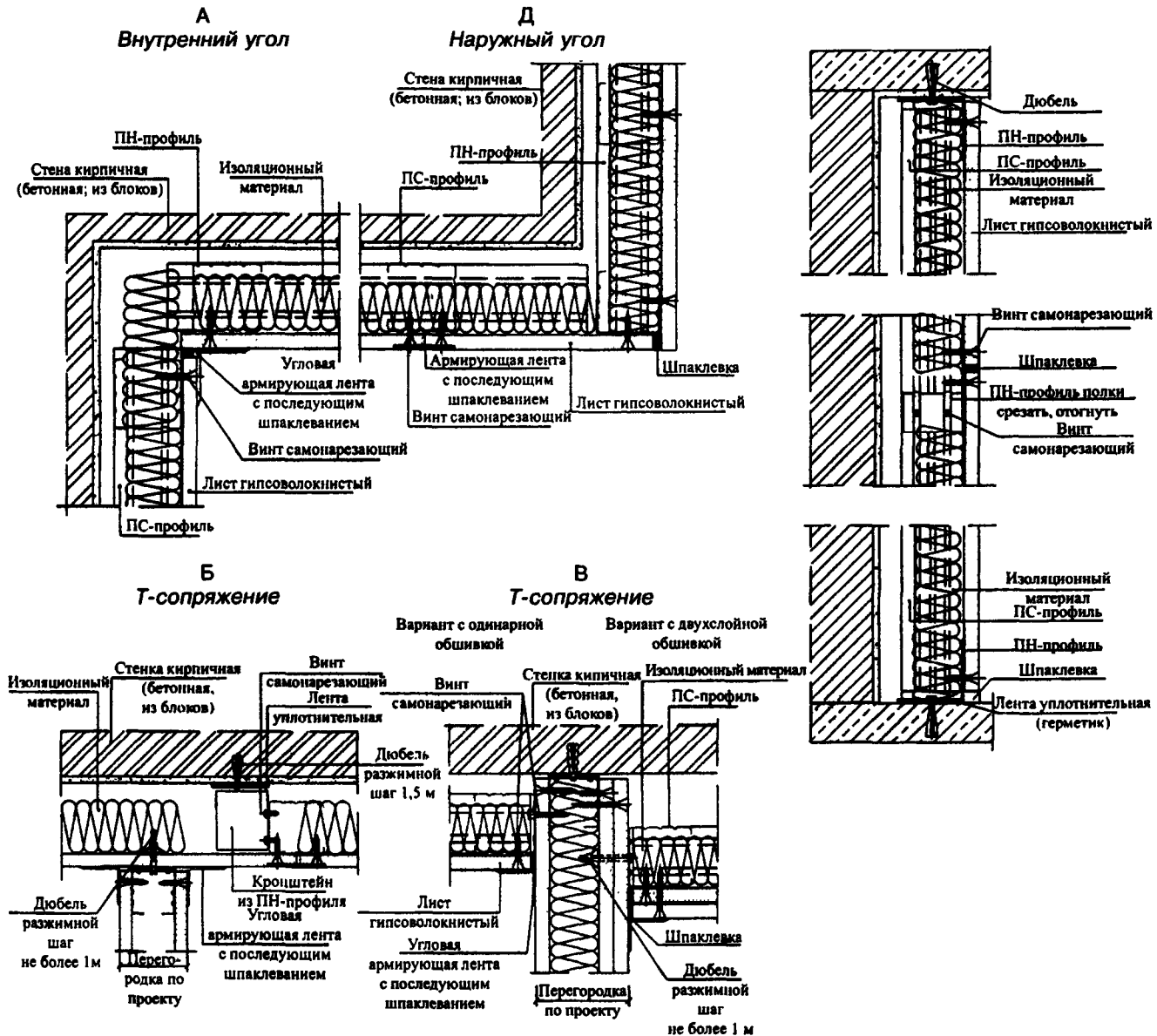
Рисунок 8 — Горизонтальный и вертикальный разрезы, узлы примыканий, внутренние и внешние углы обшивки с одинарной обшивкой гипсоволокнистыми листами по металлическому каркасу
