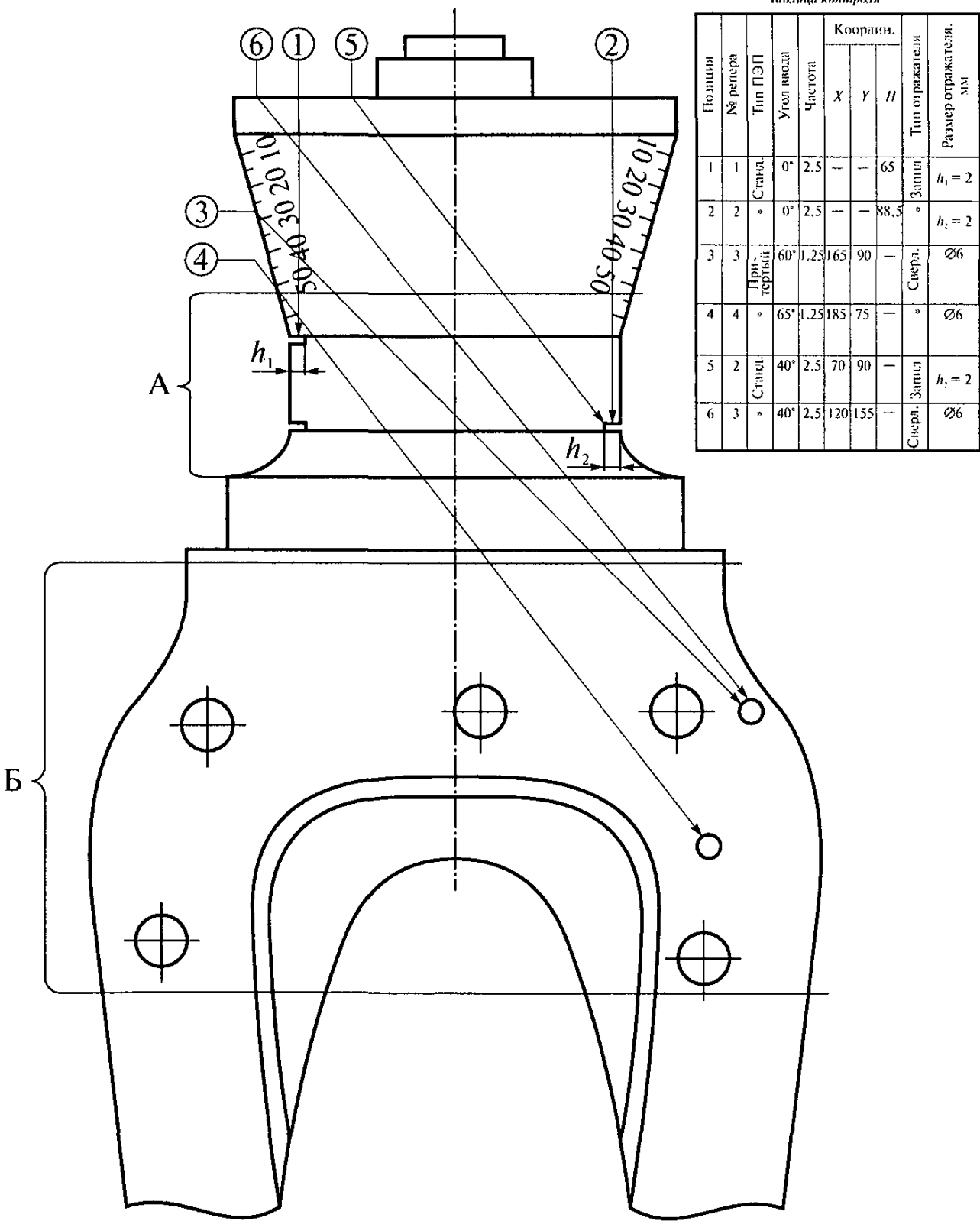
ФК4. Схема контроля лопатки ВГП типа ВОД-40
