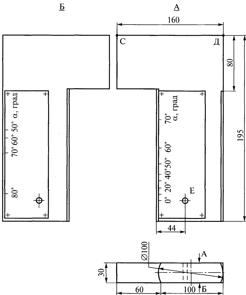
Черт. 2. Стандартный образец предприятия № 1:
