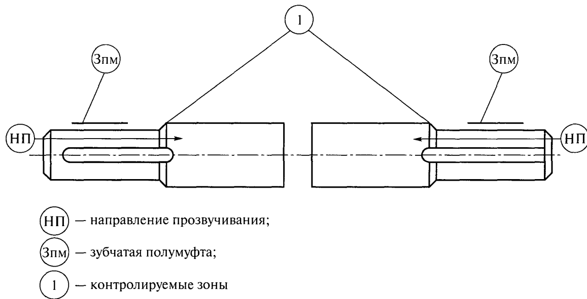
Рис. 5. Схема прозвучивания промежуточного вала
