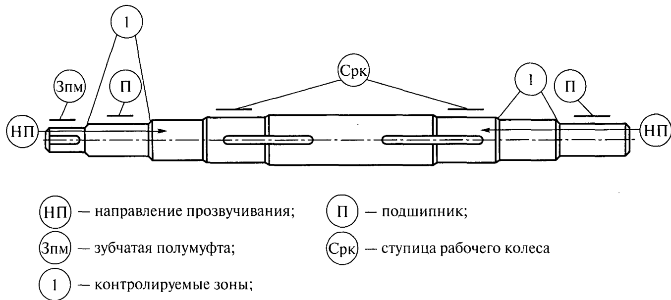
Рис. 4. Схема прозвучивания вала рабочего колеса
