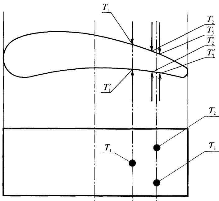
Рис. 6. Схема контроля лопатки центробежного вентилятора:
