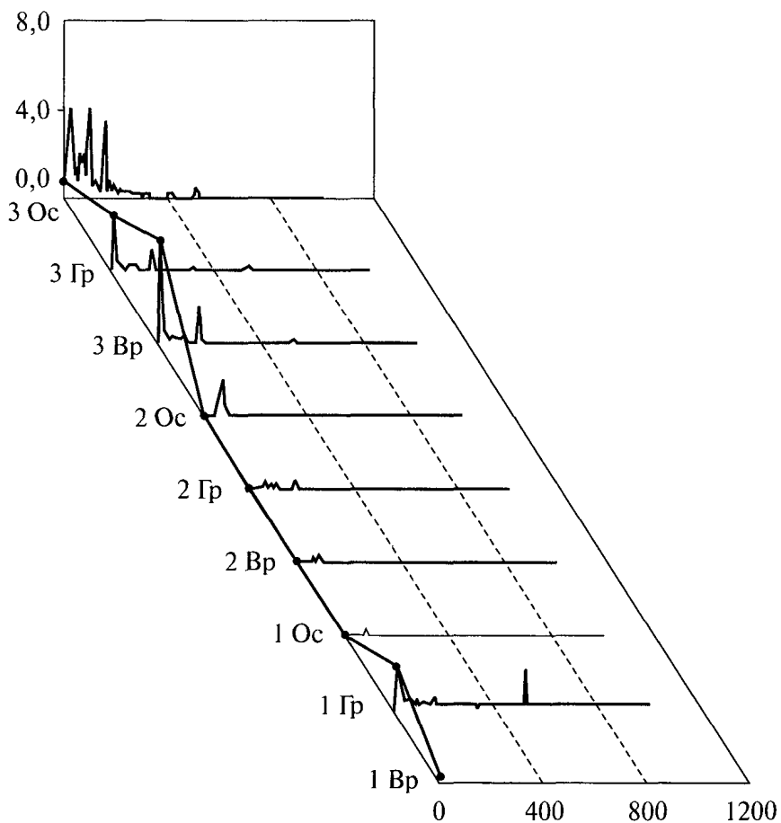
Рис. 1. Спектры механических колебаний опор электродвигателя и вентилятора
