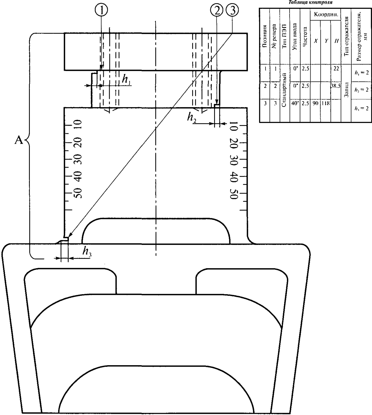
ФК2. Схема контроля лопатки ВГП типа ВОД-40М
