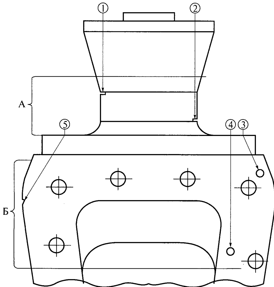
ФКЗ. Схема контроля лопатки ВГП типа ВОКД-3,6
