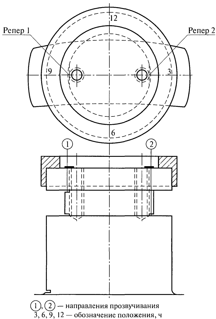
Черт. 6. Применение ограничительного кольца для УЗК цилиндрического хвостовика
