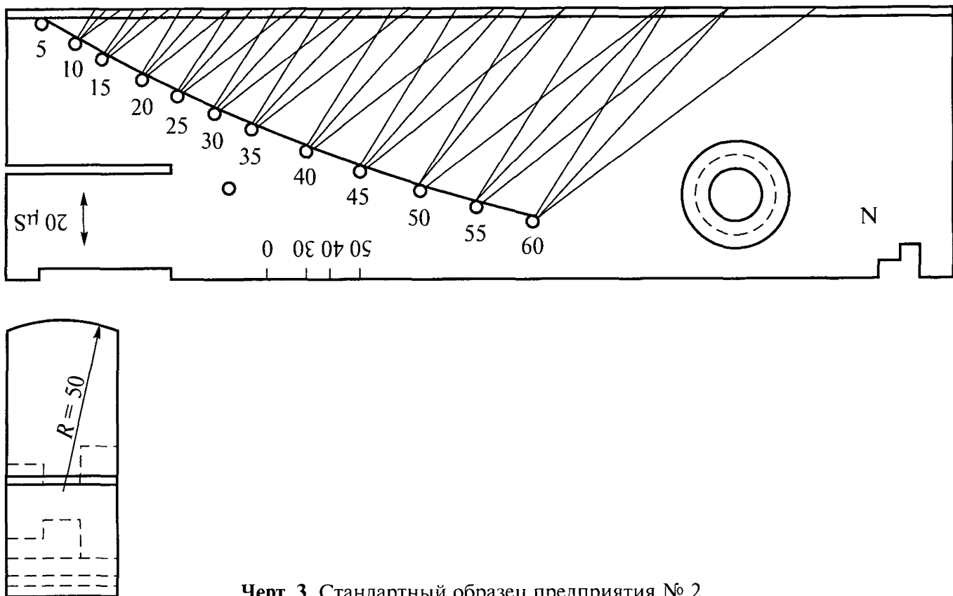
Черт. 3. Стандартный образец предприятия № 2
