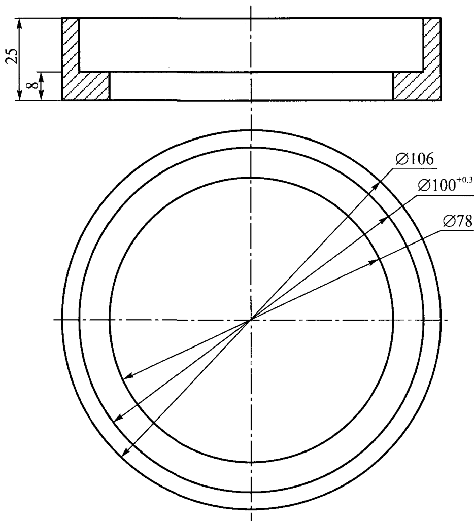
Черт. 5. Ограничительное кольцо. Материал — Ст3
