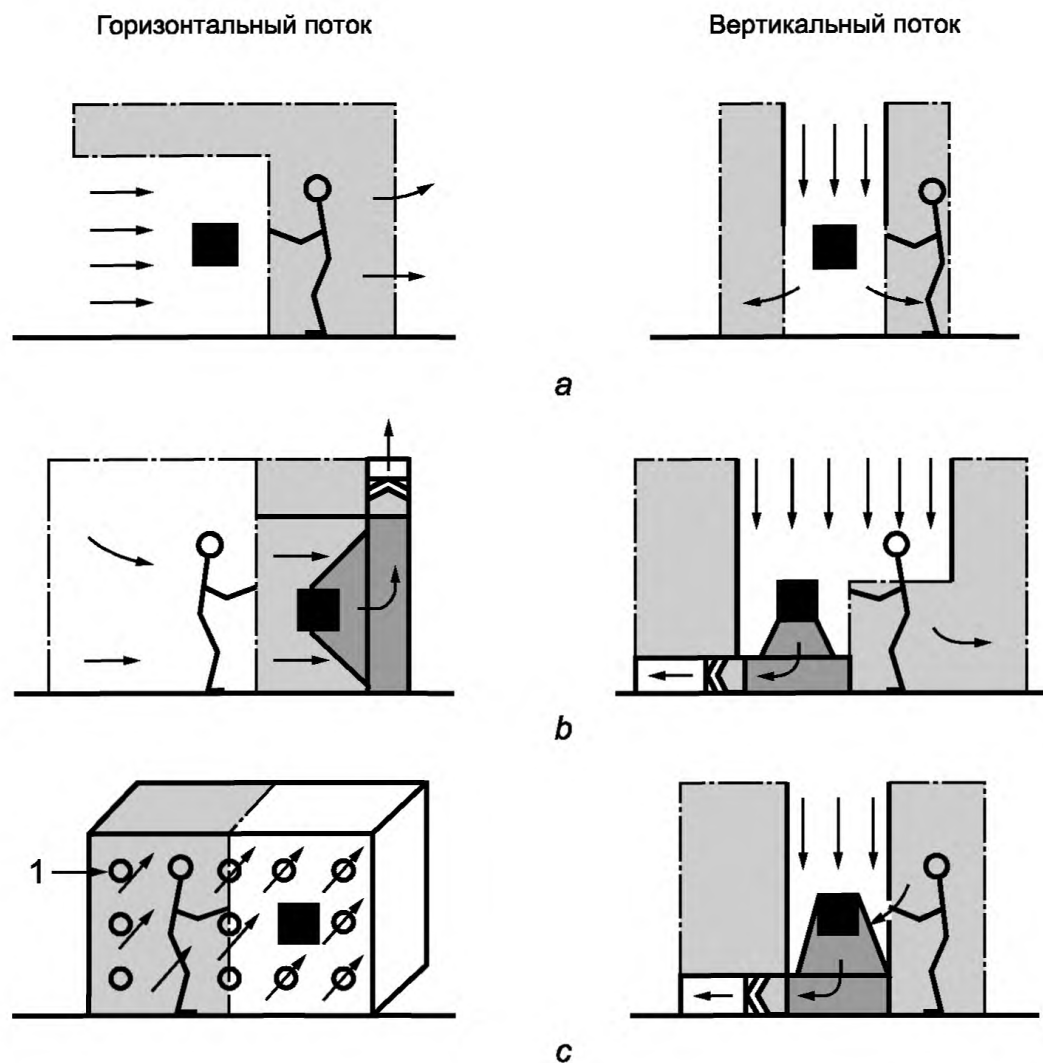
a — защита продукта; b — защита персонала и окружающей среды; c — защита персонала, продукта и окружающей среды; 1 — направление потока перпендикулярно к плоскости рисунка
