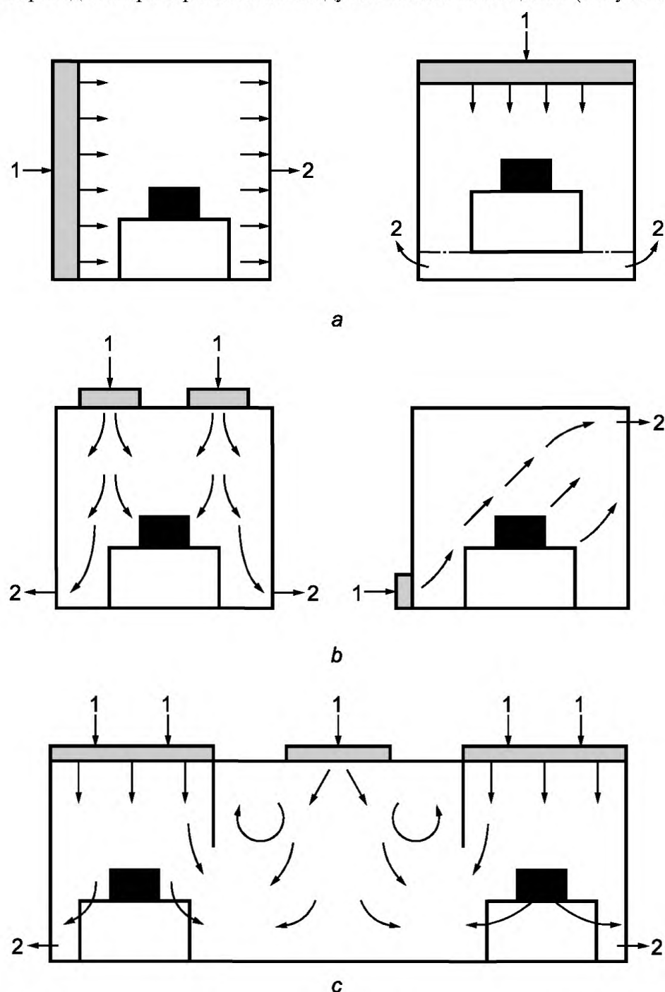
а — односторонний поток воздуха; б — неодносторонний поток воздуха; в — смешанный поток воздуха; 1 — приточный воздух; 2 — вытяжной воздух
