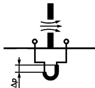
Рисунок А.7 — Принцип перепада давления
