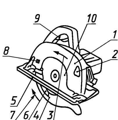
Рисунок 101 — Дисковая пила с наружным качающимся защитным кожухом
