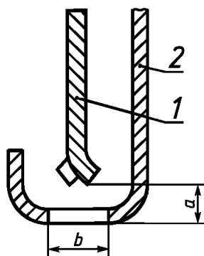
1 — пильный диск; 2 — подвижный защитный кожух
