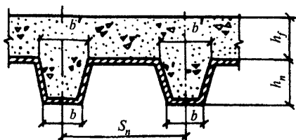
Рис. 4. К определению приведенной толщины бетона
