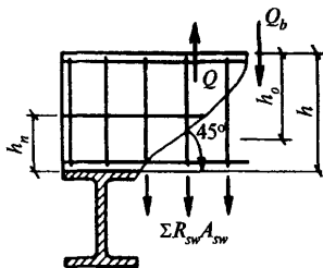
Рис. 13. Схема усилий в наклонном сечении плиты при расчете его прочности на действие поперечной силы
