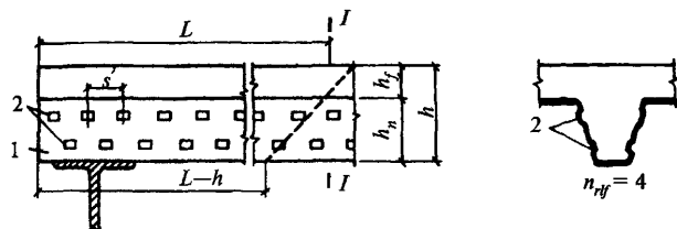
Рис. 16. Расположение рифов на стенках СПН по его концам 1 — I — сечение по пролету настила в месте наибольшего изгибающего момента, в четверти пролета, в местах приложения сосредоточенных сил; I — стальной профилированный настил; 2 — выштампованные рифы; L — длина участка расположения рифов на стенках настила, учитываемых в расчете его анкеровки по формуле (23)
