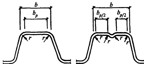
Рис. 5. К определению ширины плоских участков сжатых полок
