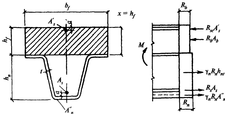
Рис. 12. Схема усилий в пролетном сечении плиты при расположении нейтральной оси в полке СПН
