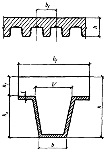
Рис. 9. Расчетное сечение плиты в пролете (выштампованные рифы в сечении условно не показаны)
