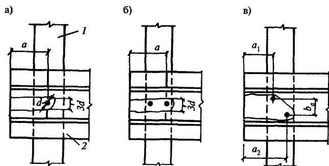
Рис. 15. К определению l'_{an} 1 — балка; 2 — настил; d — диаметр анкера (для случаев а и б l'_{an} = 2a + 3d ; для случая в l'_{an} = a_1 + a_2 + b_a + 3d )
