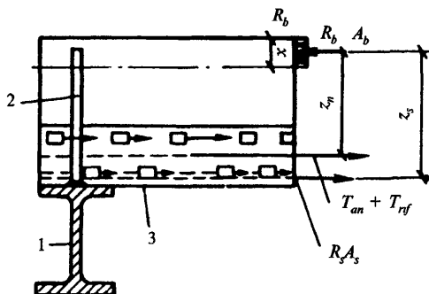
Рис. 14. Схема усилий при расчете по прочности анкеровки
