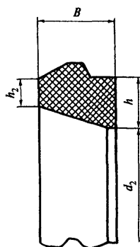
Рисунок 5 — Резиновое кольцо (размеры по таблице 8)
