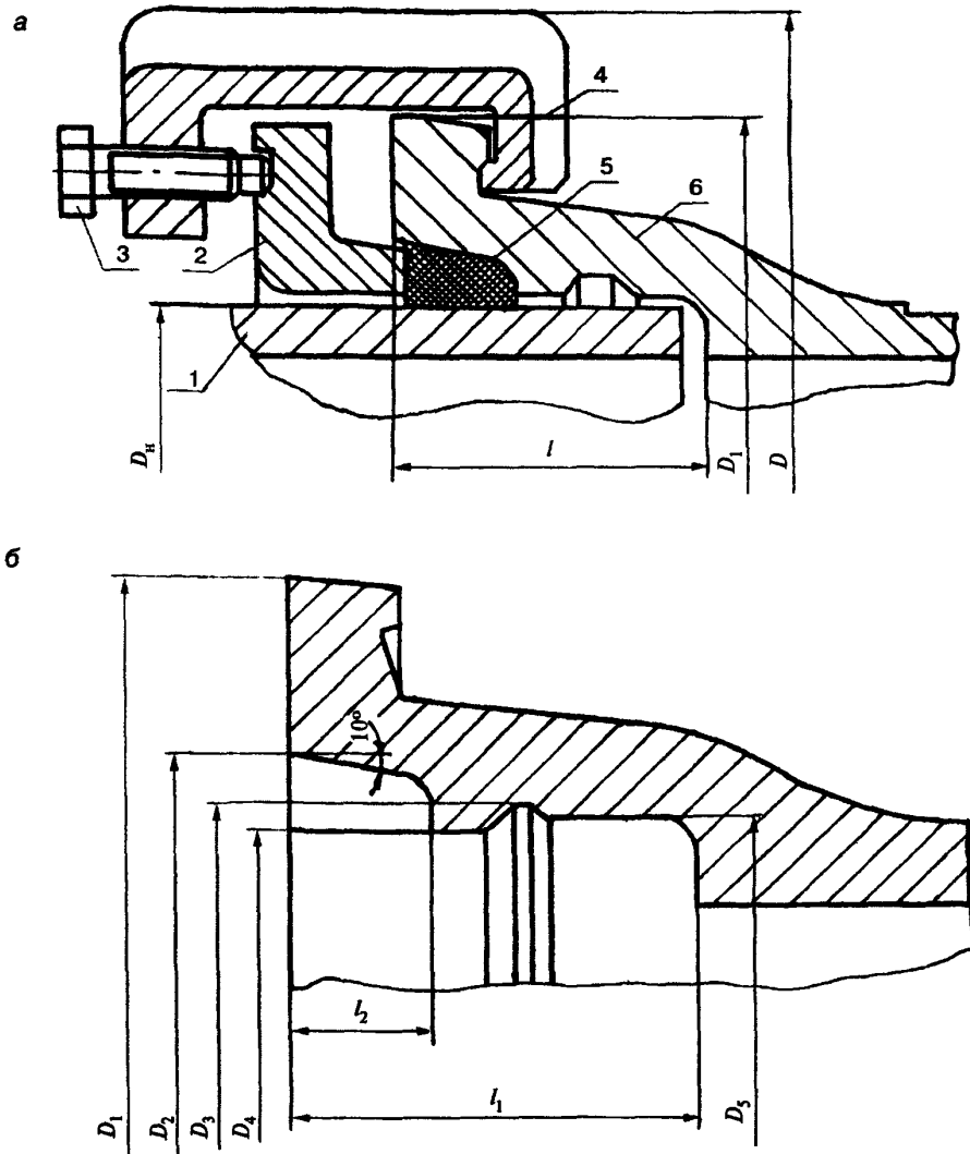
а — раструбное соединение; б — раструб трубы с резиновым кольцом
