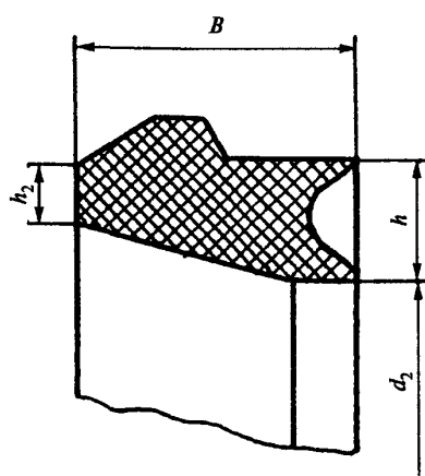
Рисунок 7 — Резиновое кольцо (размеры по таблице 10)
