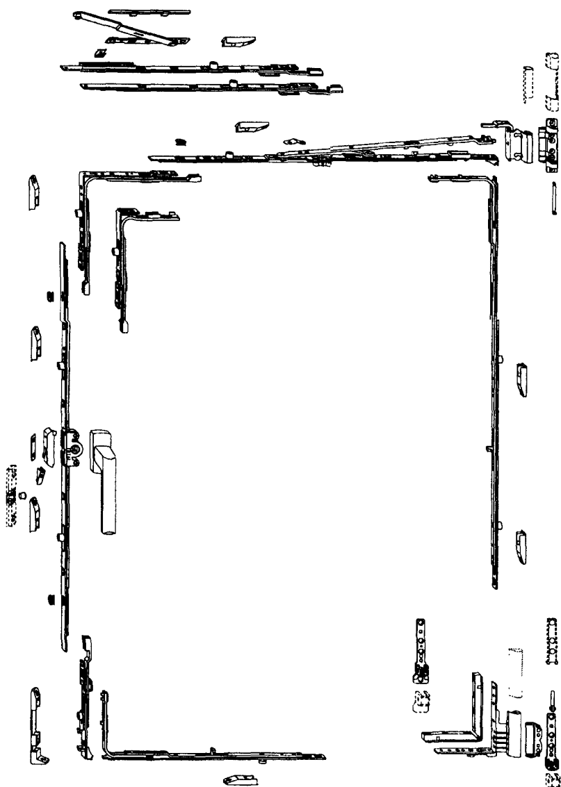
Рисунок Б.3 — Устройство поворотно-откидное
