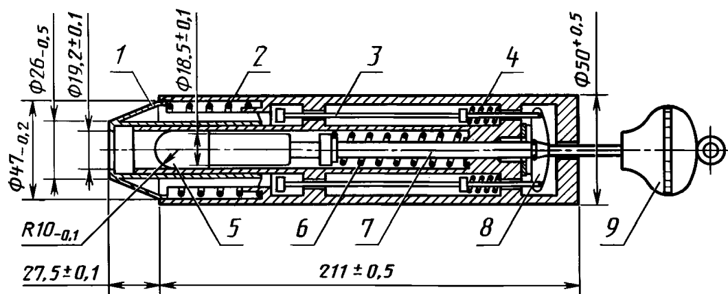
Устройство для испытания на удар
