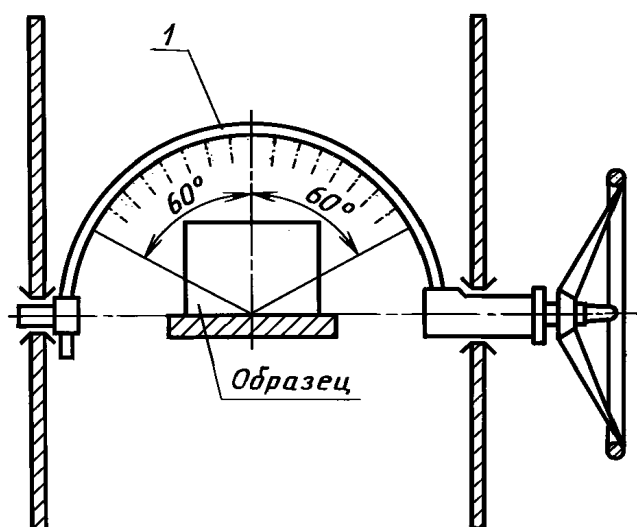
Устройство для испытания наклонным дождем
