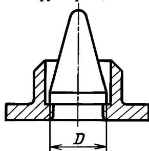
Устройство для испытания буртиков во вводах трубопроводов
