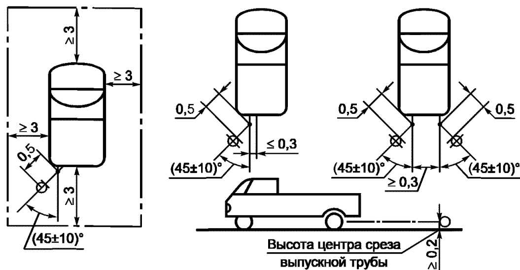
Рисунок 3.2 — Положения неподвижных транспортных средств при измерениях
