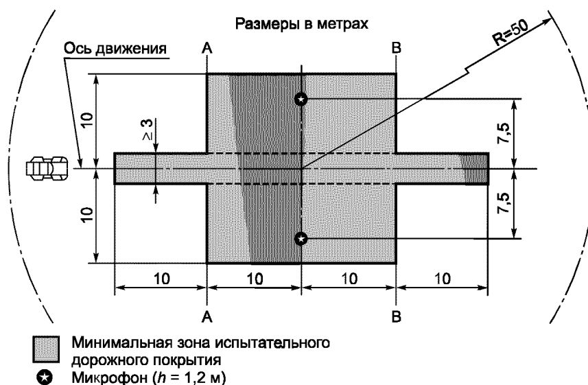
Рисунок 4.1 — Минимальные требования к зоне с испытательным дорожным покрытием
