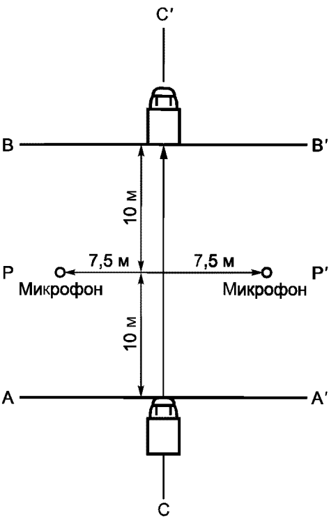
Рисунок 3.1 — Положения движущихся транспортных средств при измерениях
