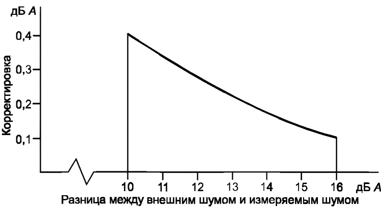
Рисунок 3.1а — Диаграмма корректировки уровня шума
