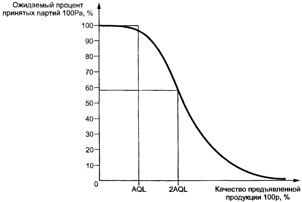
Рисунок 9 — Оперативная характеристика для плана выборочного контроля, имеющего высокую вероятность приемки при любой партии с качеством лучше AQL
