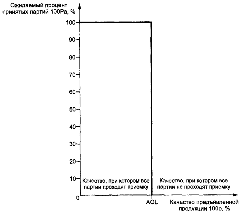
Рисунок 7 — Идеальная кривая оперативной характеристики
