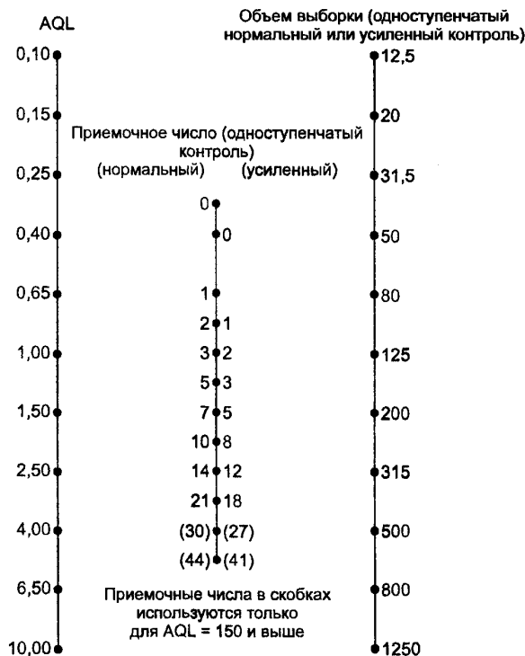
Рисунок 12 — Номограмма для метода отбора выборок, кода и объема выборки в ГОСТ Р 50779.71
