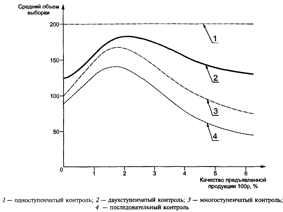
Рисунок 5 — Сравнение средних объемов выборки для планов одно-, двух-, многоступенчатого и последовательного контроля (для приемочных планов из рисунка 4)
