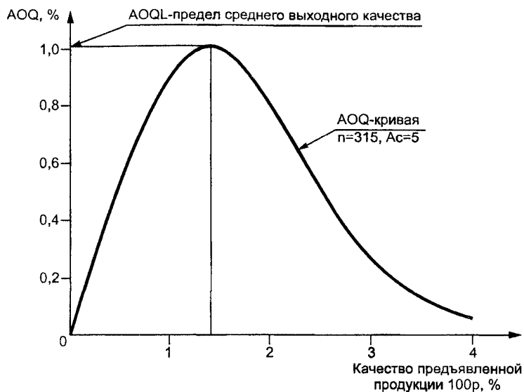
Рисунок 1 — AOQ и его предел AOQL
