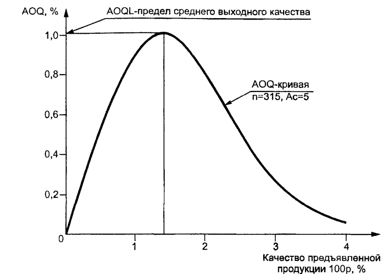
Рисунок 1 — AOQ и его предел AOQL
