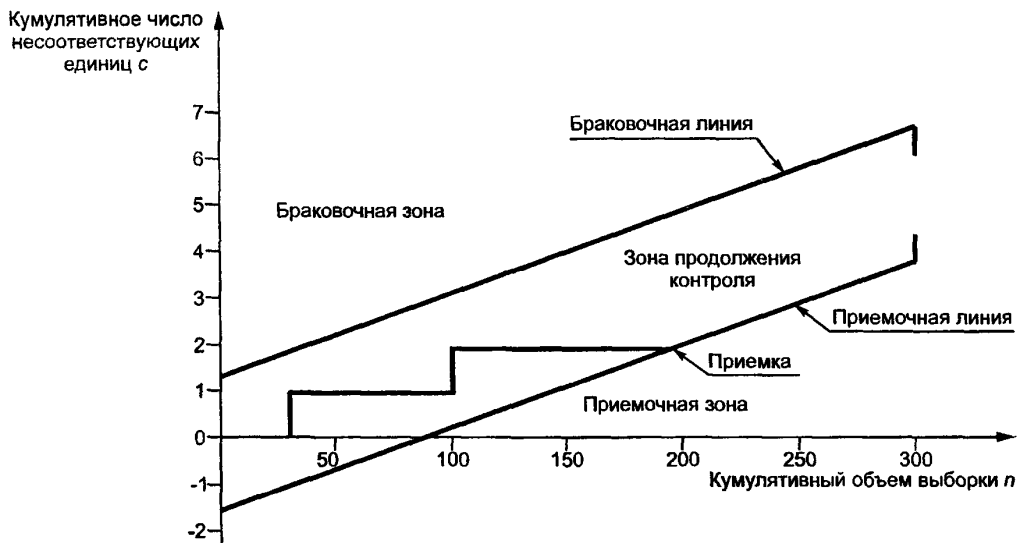
Рисунок 3 — Работа с выборочным планом усеченного последовательного контроля с AQL = 0,65\% и кодом объема выборки L
