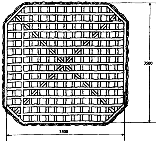
Конструкция ПСН
