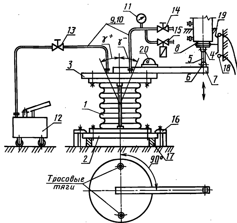
Испытание СК сдвигово-поворотного типа по подтверждению вероятности безотказной работы при изгибе (повороте)
