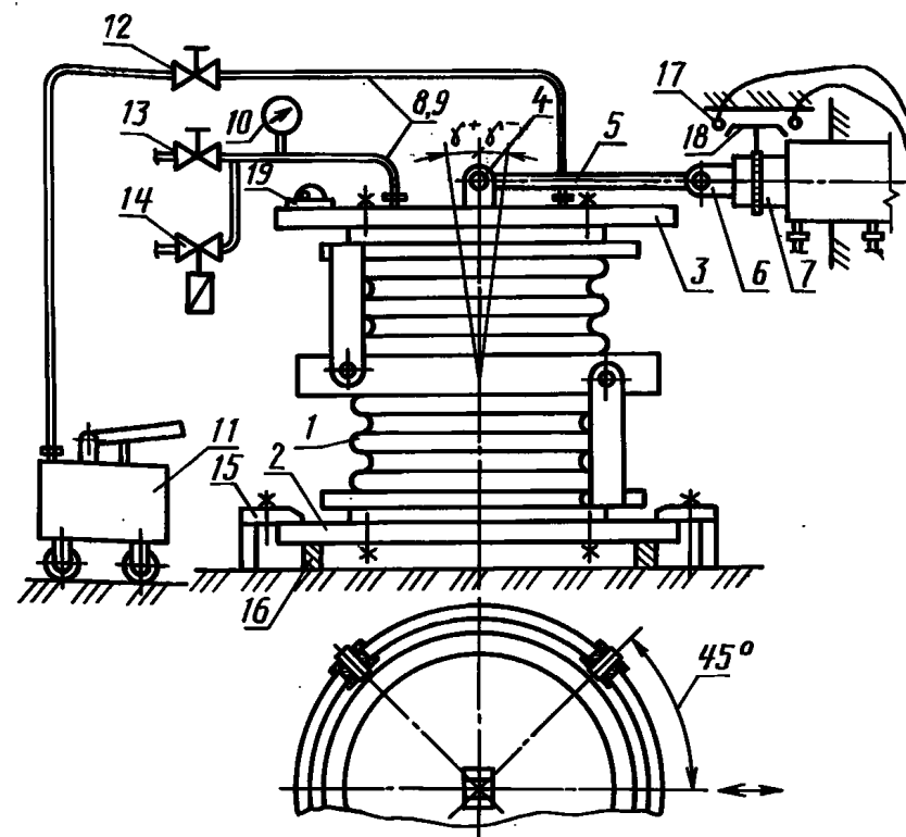
Испытание по подтверждению вероятности безотказной работы сильфонных компенсаторов поворотного типа
