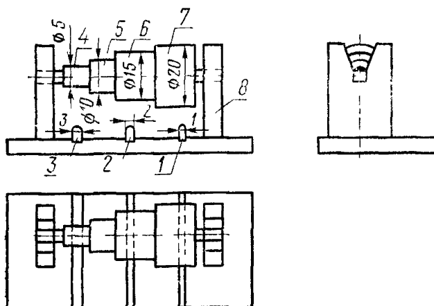
1 — 7 — стержни; 8 — стойка
