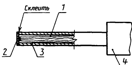
Щуп для измерения температуры поверхности
