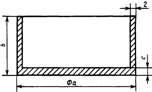
Стандартный испытательный сосуд для нагревательных элементов
