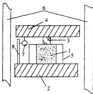
Рис. 11.7. Схема испытания на глубину вдавливания штампа: 1 – образец; 2, 4 – нижняя и верхняя плиты прессы; 3 – штамп круглый; 5 – емкость для термостатирования; 6 – штанги; 7 – индикатор; 8 – стойка
