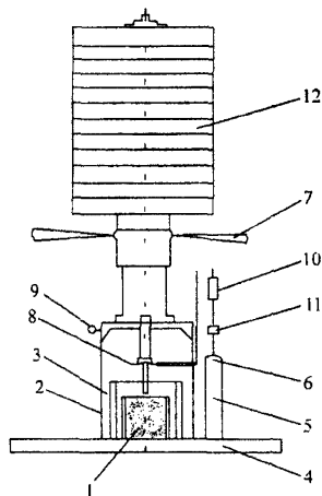
Рис. 11.6. Прибор для определения глубины вдавливания штампа: 1 – образец; 2 – форма; 3 – емкость для выдерживания образца; 4 – стол прибора; 5 – круглый штамп; 6 – шарик; 7 – рукоятка; 8 – шток; 9 – контрольная лампочка; 10 – индикатор часового типа; 11 – опорный столик; 12 – грузы
