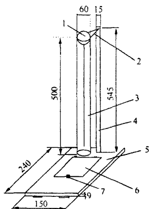
Рис. 11.10. Схема прибора для определения прочности приклепки зерен щебня к поверхности вяжущего по методу Виолит:
