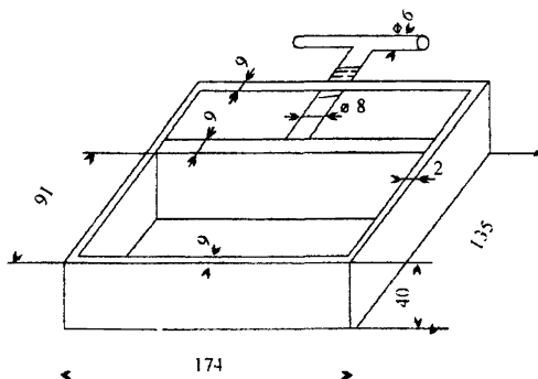
Рис. 11.3. Форма для изготовления образца шва
