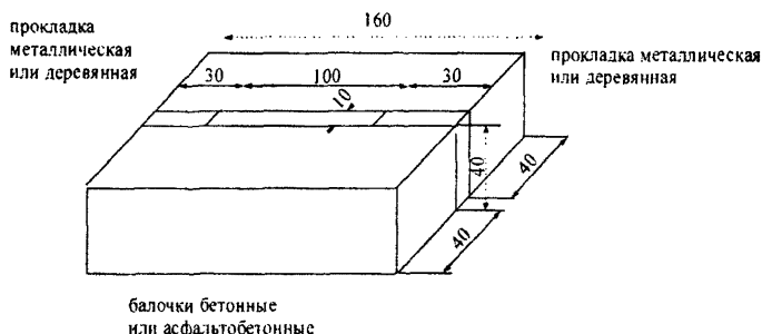
Рис. 11.4. Схема формы для испытания образца трещины
