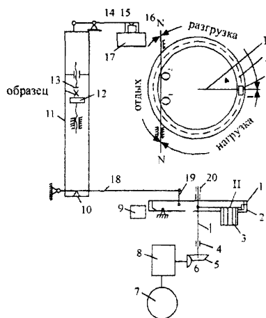
Рис. 11.8. Кинематическая схема механического рычажного пресса:
