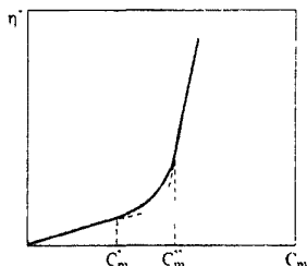
Рис. 1.1. Зависимость вязкости от концентрации фазы в КОВ
