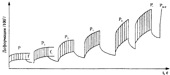
Рис. 11.9. Фотодиаграмма испытания образца асфальтобетона на изгиб при температуре 0^{\circ}\text{C} : P, P_1, \dots – возрастающие нагрузки; f, f_1 – упругий прогиб
