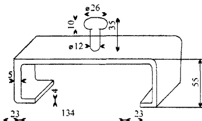
Рис. 11.2. Схема закрепления образца вяжущего
