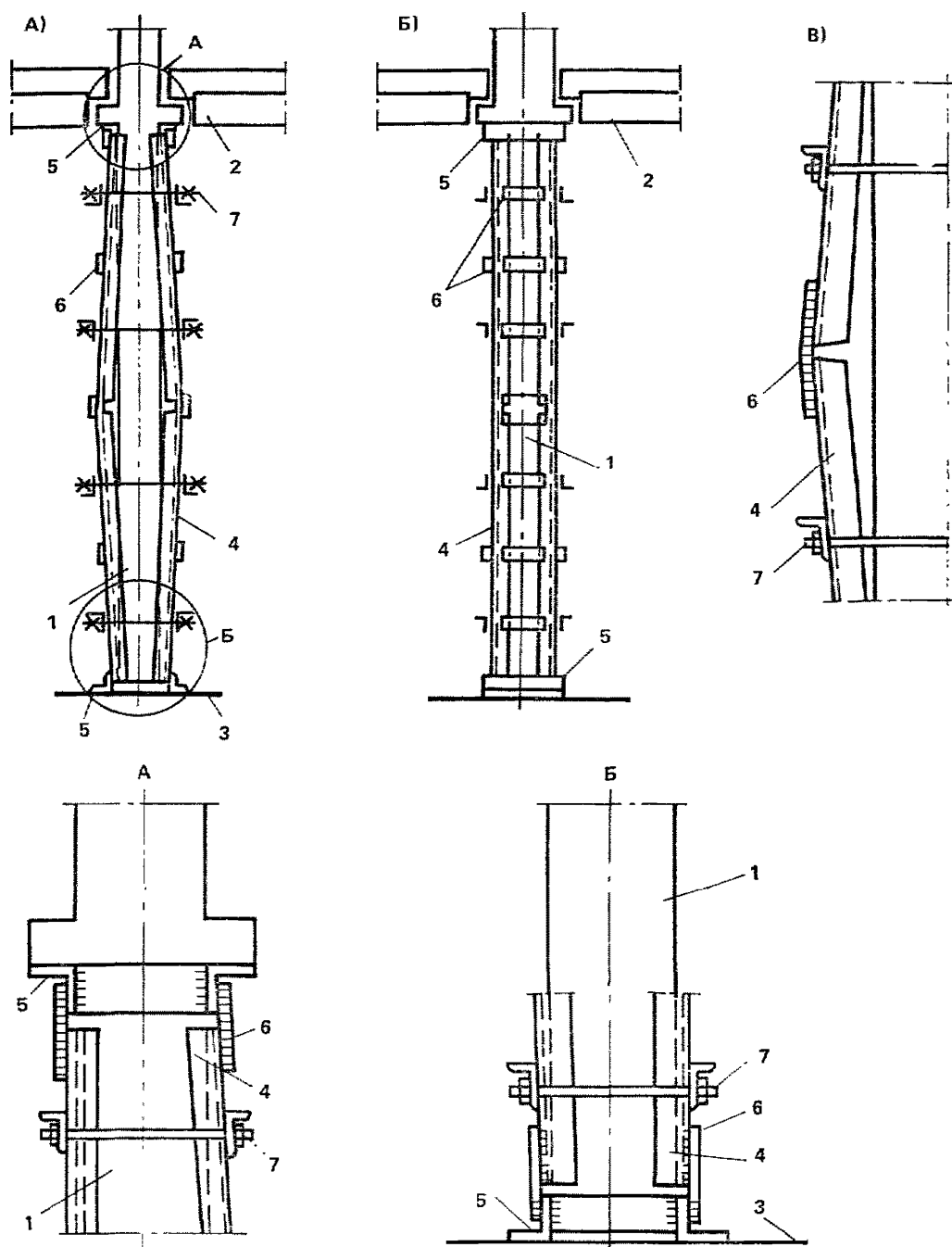
Рис. 23. Усиление колонн стальной обоймой (с преднапряжением, стягиванием ветвей или подклинкой)
