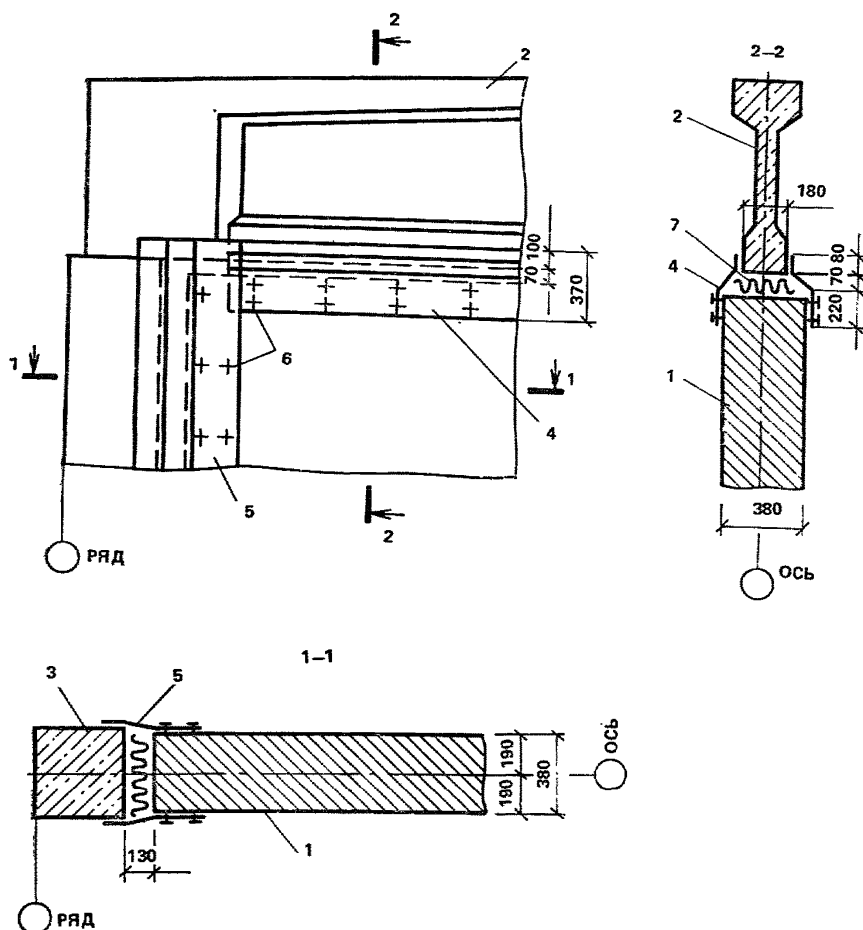
Рис. 37. Устройство зазора между железобетонными несущими конструкциями и внутренней кирпичной стеной
