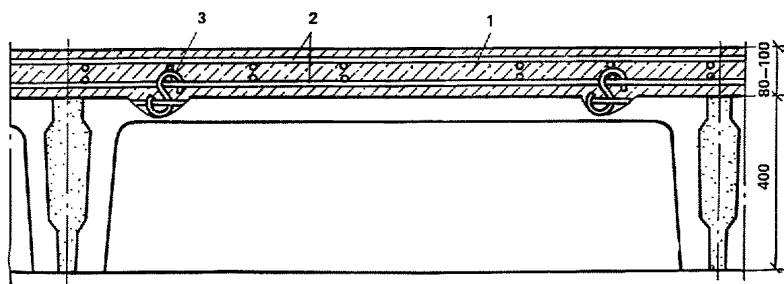
Рис. 3. Усиление ребристых плит перекрытий многоэтажных производственных зданий
