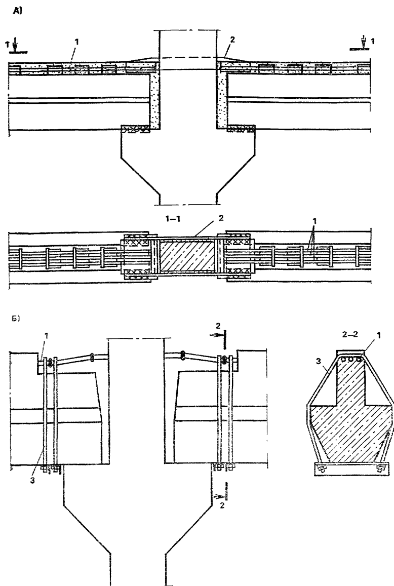
Рис. 34. Усиление узловых сопряжений ригелей с колоннами каркасов многоэтажных производственных зданий при разрыве или искривлении надопорных стержней
