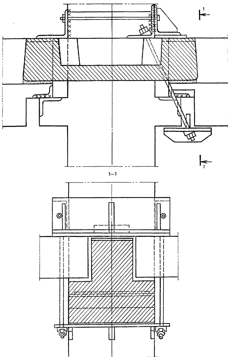
← Рис. 35. Усиление узловых сопряжений ригелей с колоннами рамно-связевых каркасов наращиванием опорной закладной детали ригеля
