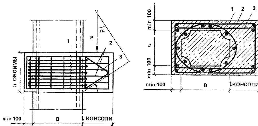
Рис. 26. Осуществление новых консолей (упоров) с устройством обоймы на стволе колонны
