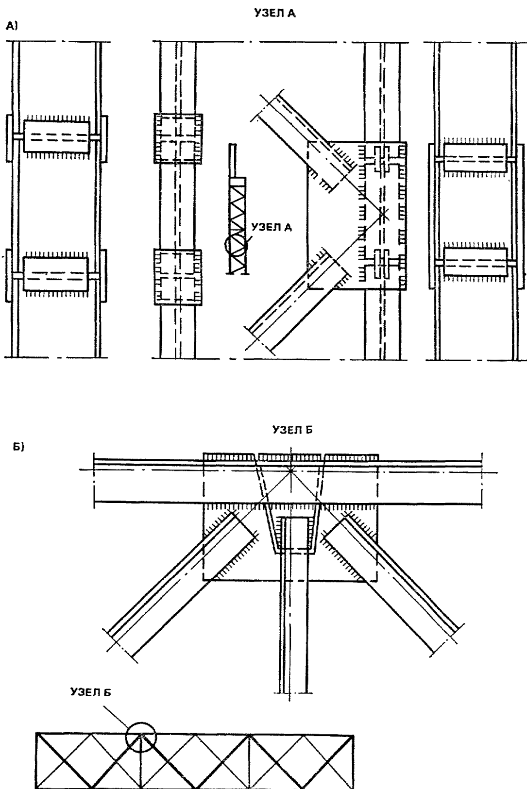
Рис. 56. Примеры восстановления А — колонны — заменой поврежденных частей; Б — ферм — устройством второй решетки (жирными линиями показаны новые раскосы и фасонки)
