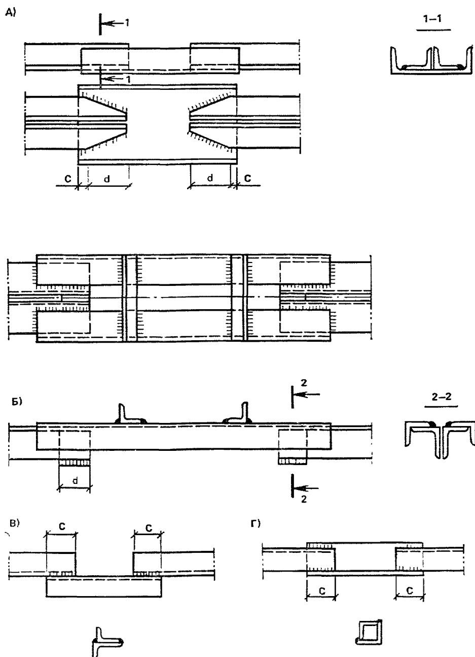
Рис. 50. Восстановление элементов ферм вырезанием и заменой поврежденной части
