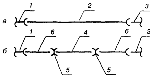
а — до ремонта, б — после ремонта 1, 3 — деталь трубопровода, 2 — поврежденный патрубок, 4 — патрубок без раструба, 5 — надвижная муфта, 6 — неповрежденные участки патрубка 2
