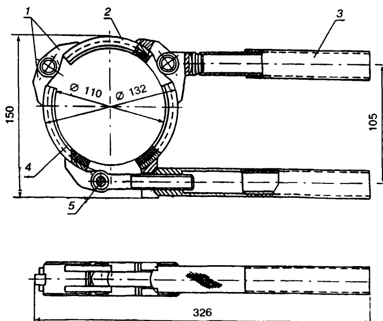
Рисунок 12 — Соединение гладкого конца детали из ПП с чугунным раструбом
