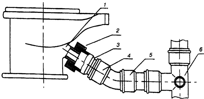
Рисунок 9 — Резиновая манжета для присоединения пластмассового сифона
