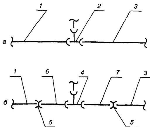
а — до ремонта; б — после ремонта 1, 3 — патрубок, 2 — поврежденная фасонная часть, 4 — новая фасонная часть, установленная взамен поврежденной, 5 — надвижная муфта, 6 — патрубок с раструбом, 7 — патрубок без раструба
