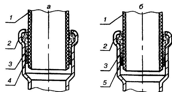
Рисунок 11 — Резиновая манжета для присоединения унитаза
