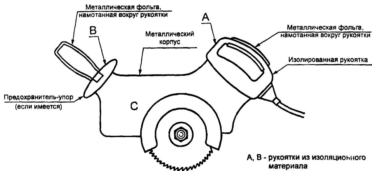
Рисунок 8в — Ручная (портативная) электропила
