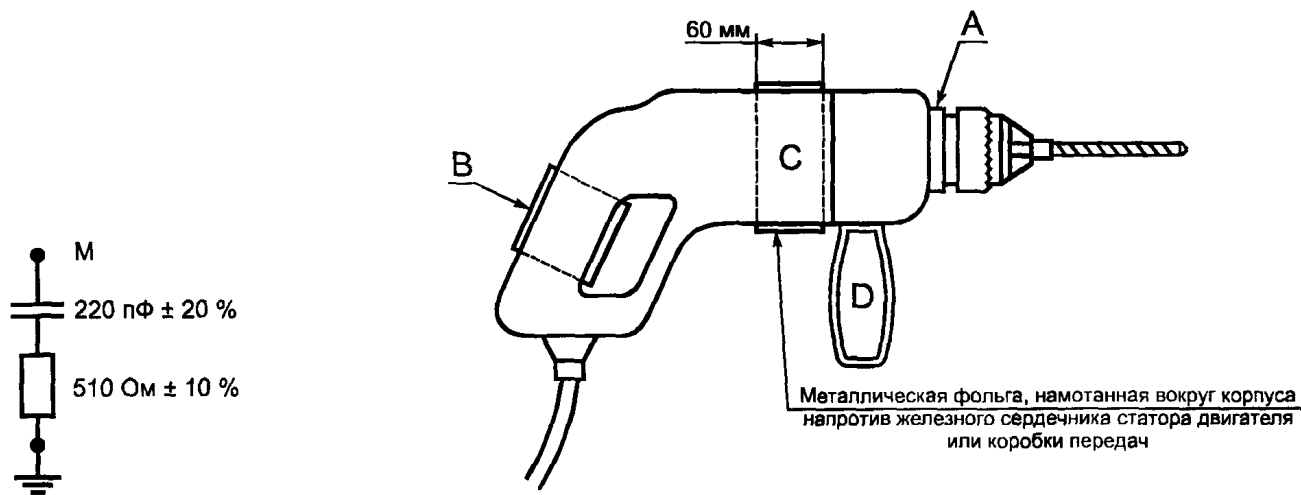
Рисунок 8а — Элемент RC
