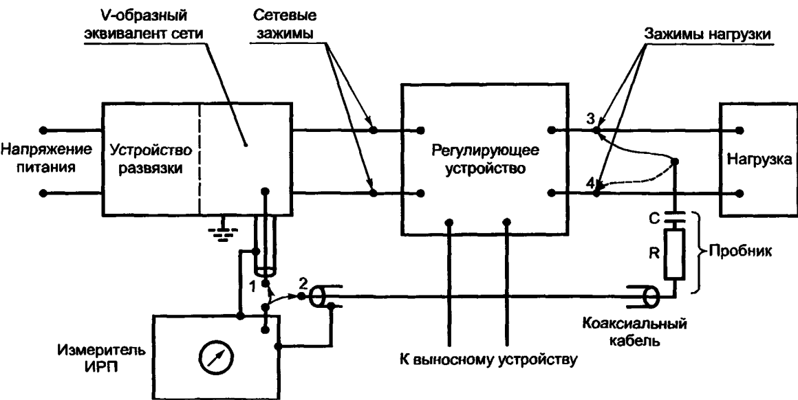
1 — положение переключателя при измерениях на сетевых зажимах; 2 — положение переключателя при измерениях на зажимах нагрузки; 3, 4 — наиболее приемлемые соединения во время измерений; C — конденсатор пробника ( C \geq 0,005 \text{ мкФ} ); R — резистор пробника ( R \geq 1500 \text{ Ом} )
