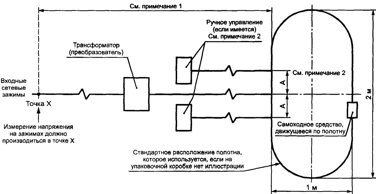
Рисунок 6 — Схема измерения напряжений ИРП, создаваемых на зажимах устройств питания электрических ограждений
