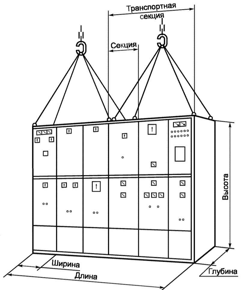
Рисунок С.4 — НКУ заводского изготовления много-шкафного типа
