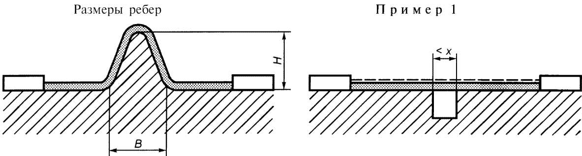
B — минимальная ширина основания согласно требованиям к механической прочности; H — минимальная высота 2 мм
