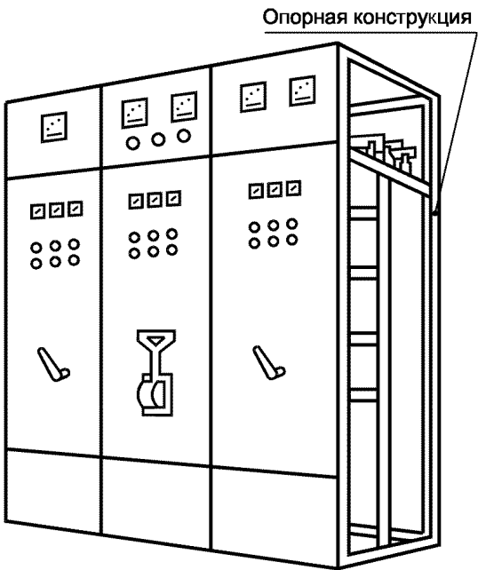
Рисунок С.2 — НКУ заводского изготовления открытого типа, защищенное спереди
