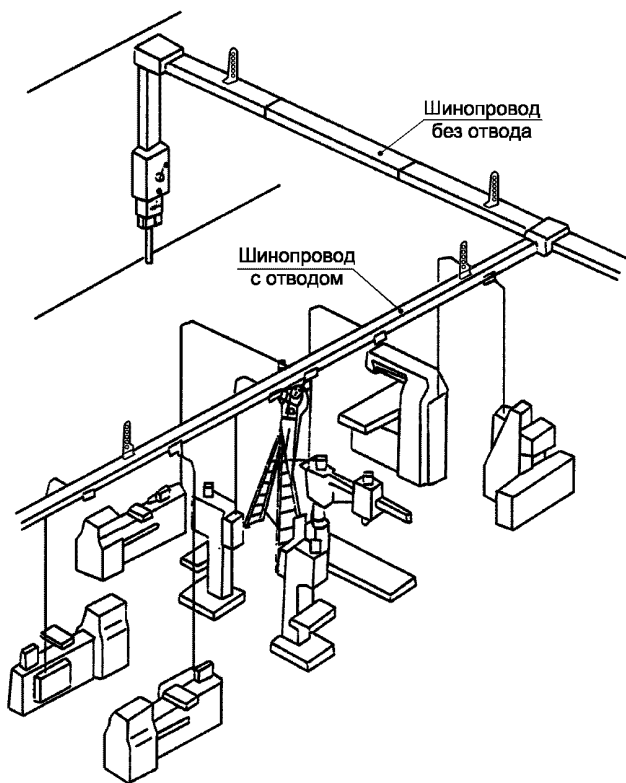
Рисунок С.7 — Система сборных шин (шинопровод)
