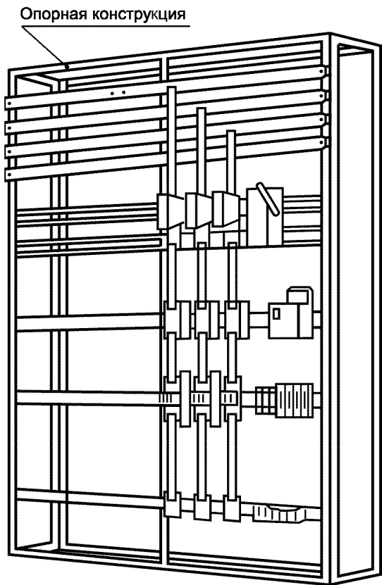
Рисунок С.1 — НКУ заводского изготовления открытого типа
