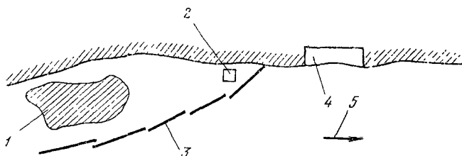
Рис. 15. Каскадное расположение бон: 1 — нефтяное пятно; 2 — нефтеприемник; 3 — бон; 4 — защищаемый объект; 5 — направление течения
