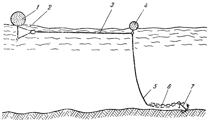
Рис. 21 Установка бонового заграждения на буй 1 — буй; 2 — оттяжка бона, 3 — синтетический канат, 4 — буй; 5 — канат буй, 6 — якорь-цепь, 7 — якорь
