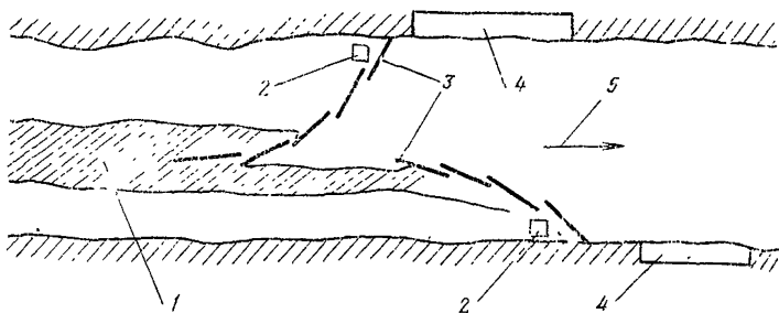
Рис. 14. Шевронное расположение бон: 1 — нефтяное пятно; 2 — нефтеприемник; 3 — бон; 4 — защищаемый объект; 5 — направление течения
