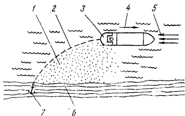
Рис. 19. Перемещение судна для увеличения ограждаемого судном и боновыми участками:
