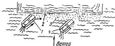
Рис. 7 Сбор загрязняющих веществ у причалов и молов
