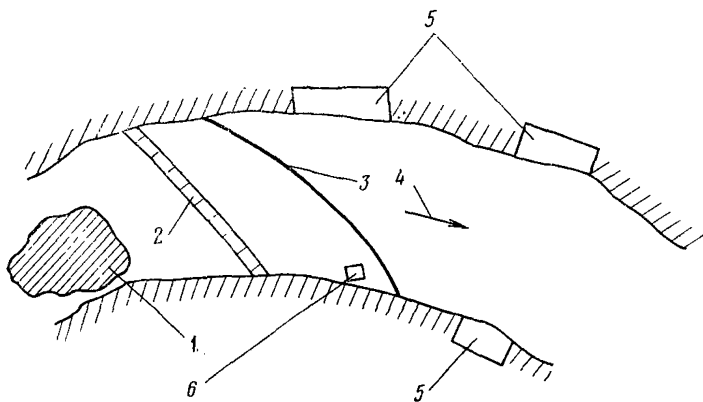
Рис. 16. Диагональное расположение бон: 1 — нефтяное пятно; 2 — защита от плавающих предметов; 3 — боновое заграждение; 4 — направление течения; 5 — защищаемые объекты; 6 — нефтесборное устройство
