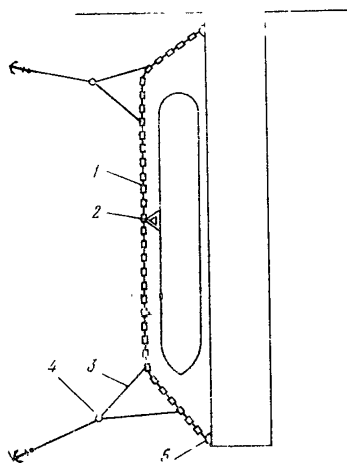
Рис 13 Ограждение бонами судна, стоящего у причала:
