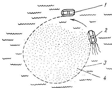
Рис. 2. Ограждение загрязненного участка открытой акватории бомами: 1 — вспомогательный нефтемусоросборщик или катер; 2 — рабочий нефтемусоросборщик; 3 — оперативные боновые заграждения; 4 — загрязняющие вещества
