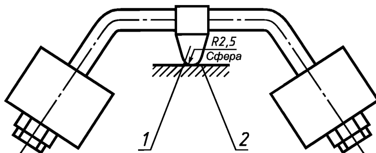
1 — стальной шарик; 2 — испытуемая поверхность
