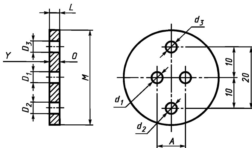
Рисунок 1 — Размеры стартеров
