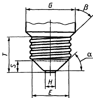
Испытательные цоколи E14 и E27
