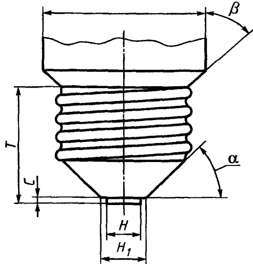
Испытательный цоколь E40
