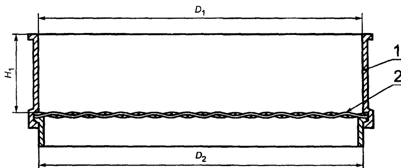
Рисунок 2 — Поперечное сечение лабораторного сита
