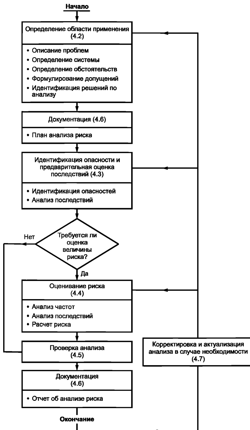
Рисунок 2 — Процесс анализа риска (раздел 4)
