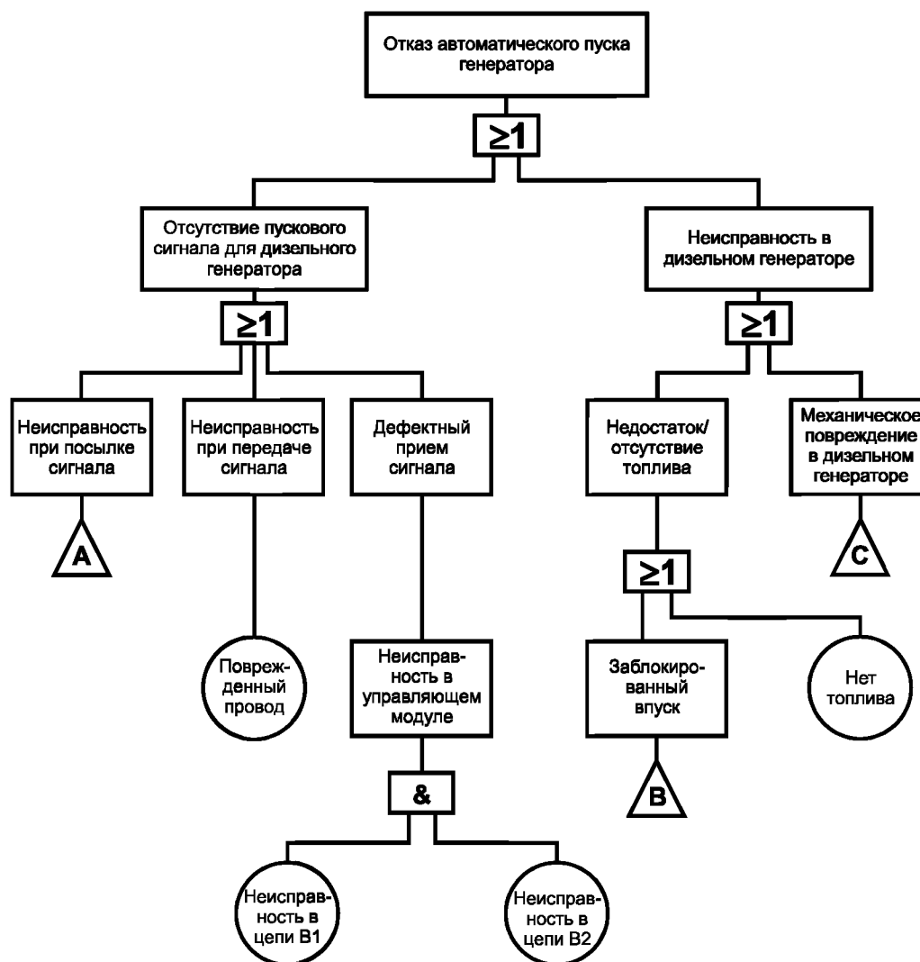
Рисунок А.1 — Пример «дерева неисправностей»
