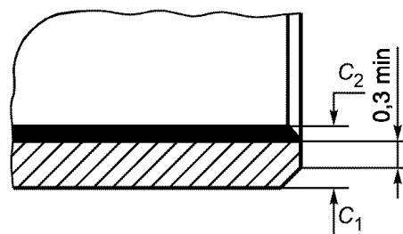
Рисунок 9 — Фаски
