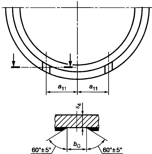
Рисунок 16 — Форма канавки на поверхности бурта
