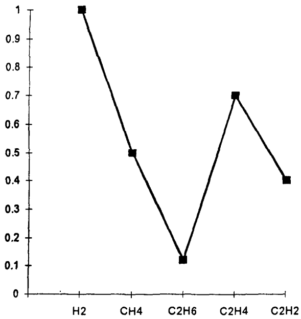
Рис. 3.3. Дефекты, вызванные искрением
