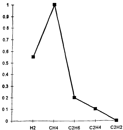
Рис. 3.8. Дефекты термического характера, переходящие в ЧР
