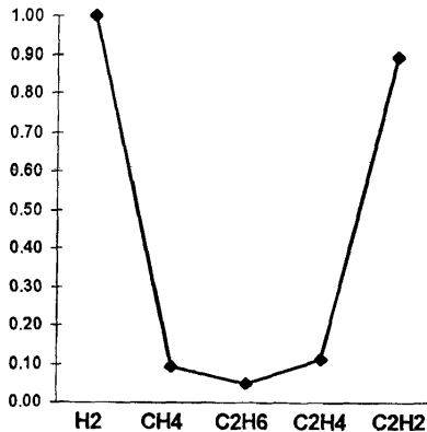
Рис.4.8 График дефекта электрического характера(дуга)
