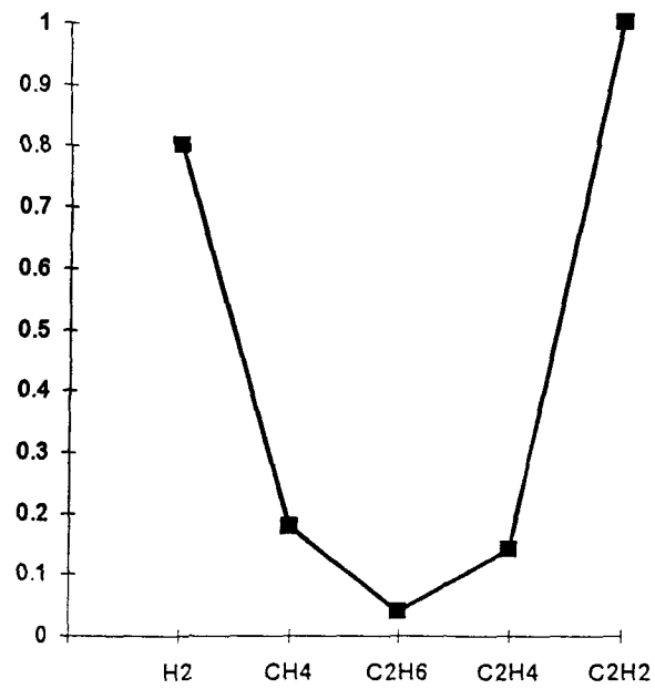
Рис. 3.5. Дефекты, вызванные дугой
