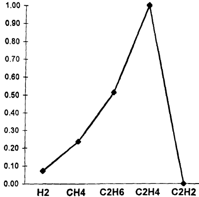
Рис.4.4. График дефекта термического характера - высокотемпературный нагрев ( >700^\circ\text{C} ), вызванный подгаром контактов переключателя
