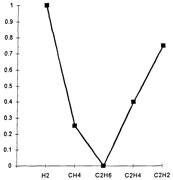
Рис. 3.4. Дефекты, вызванные дугой
