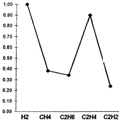
Рис. 4.7. График дефекта электрического характера (искрение)
