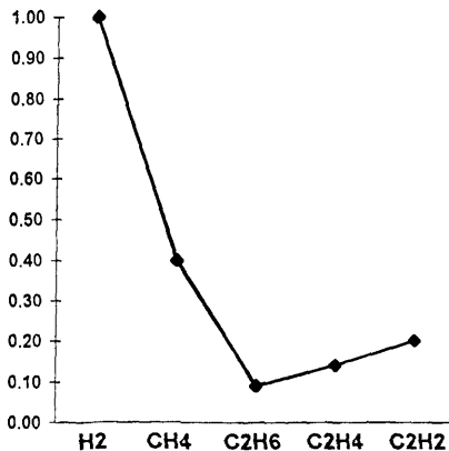
Рис.3.1. Разряды малой мощности
