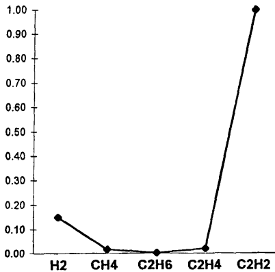
Рис.4.6. График дефекта электрического характера (дуга)
