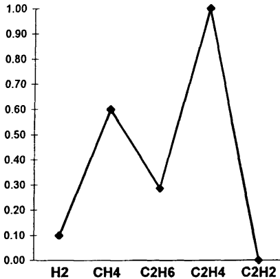
Рис. 4.3. График дефекта термического характера - высокотемпературный нагрев ( >700^{\circ}\text{C} ), вызванный касанием нижней консоли с шипом
