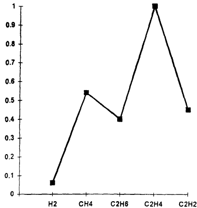
Рис.4.2. График дефекта термического характера - высокотемпературный перегрев, вызванный короткозамкнутым контуром в остоле
