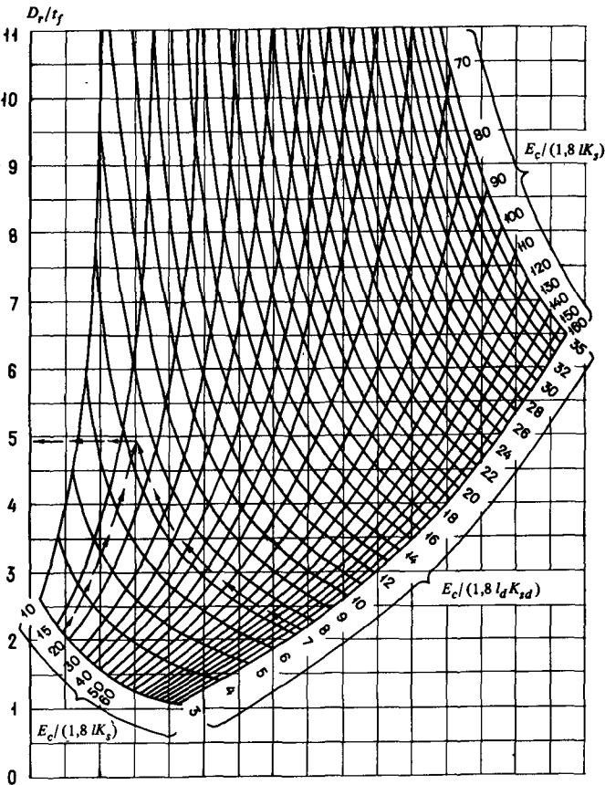
Черт. 2. Номограмма для определения соотношения \frac{D_r}{t_f}
