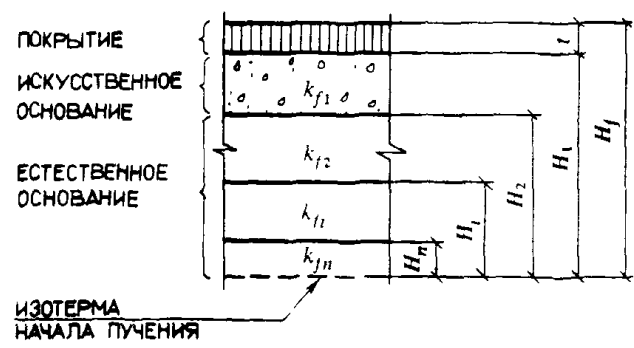
Черт. 1. Расчетная схема слоистого основания
