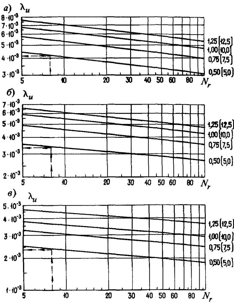
Черт. 8. График для определения предельных относительных прогибов \lambda_u , м, жестких аэродромных покрытий, устраиваемых на грунтах
