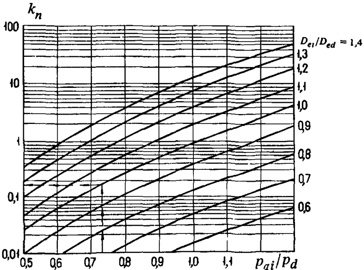
Черт. 11. Номограмма для определения коэффициентов приведения нагрузки к расчетной k_n для жестких покрытий
