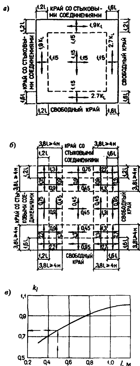
Черт. 1. Значения переходных коэффициентов k
