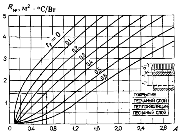
Черт. 2. Номограмма для определения термического сопротивления теплоизоляции
