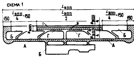
Черт. 1. Схемы деления покрытий аэродрома на группы участков
