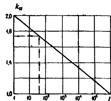
Черт. 3. График для определения коэффициента k_u
