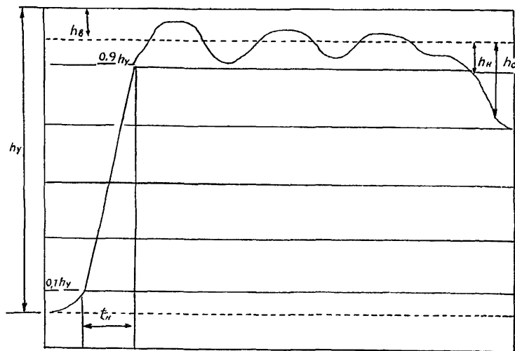
Рис. 1. Схема для определения параметров аппаратурной функции измерителя Р5-12
