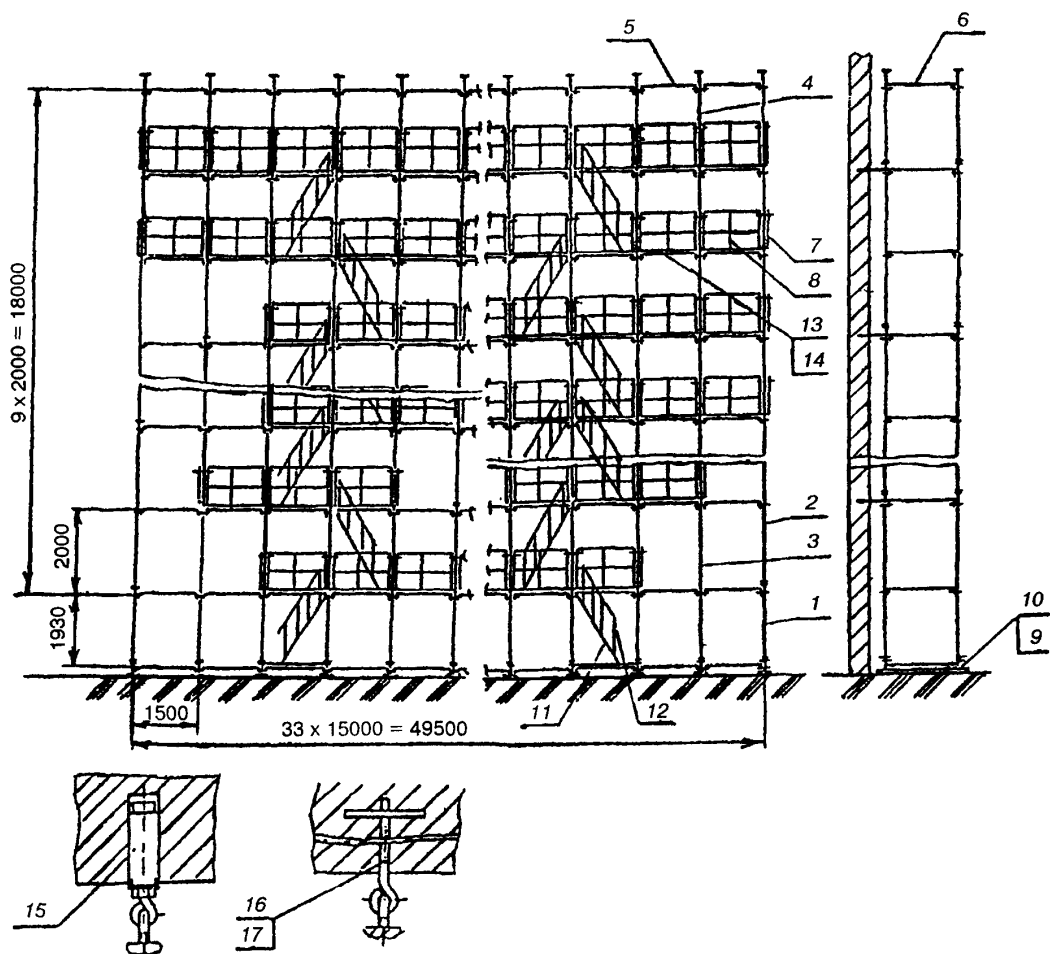
1, 2, 3, 4 — стойки; 5 и 6 — ригели; 7 и 8 — ограждения; 9 — башмак; 10 — подкладка; 11 — лестница; 12 — перила; 13 и 14 — щиты; 15 — пробка; 16 — крюк; 17 — планка
