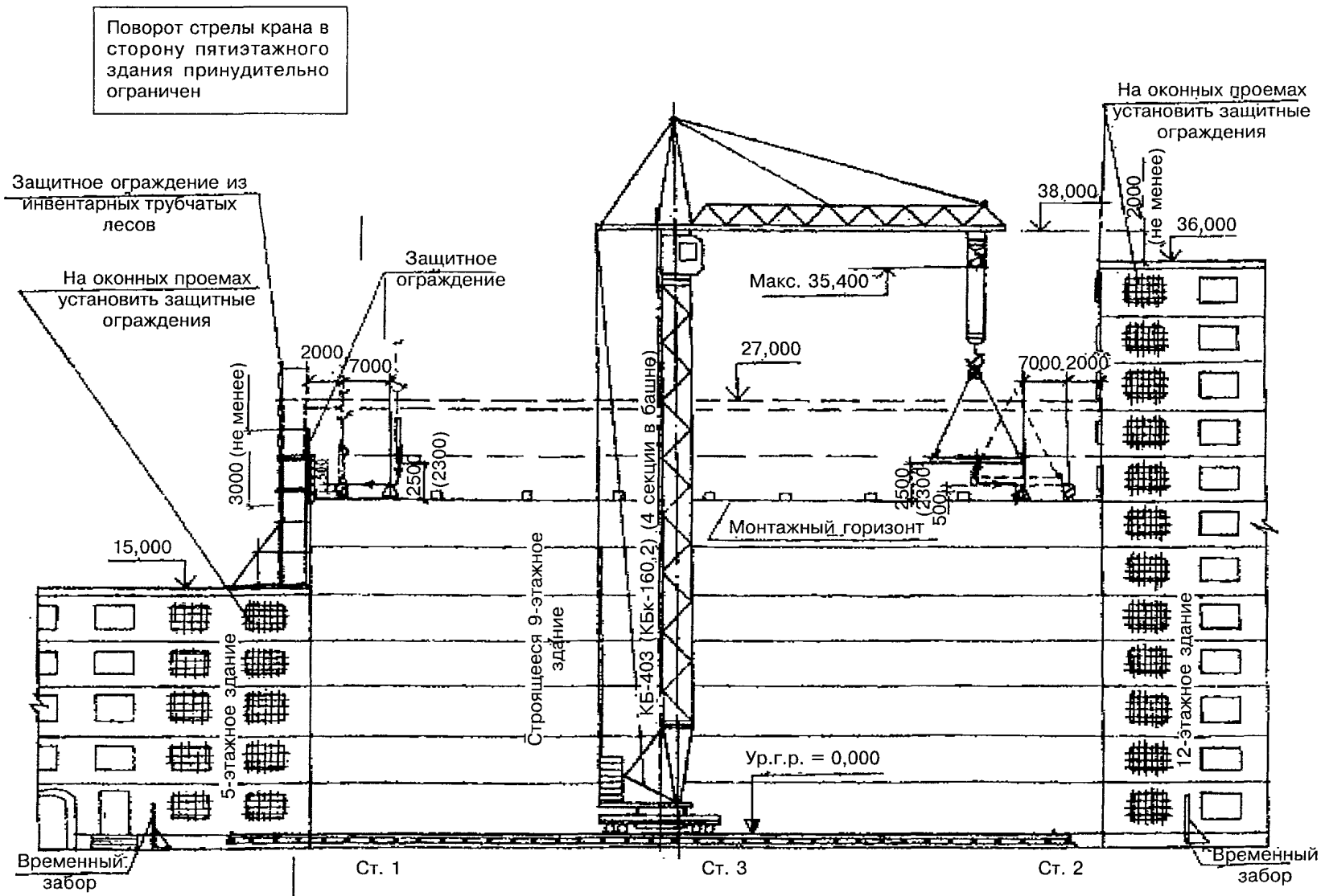
Рисунок 4 — Разрез I—I
