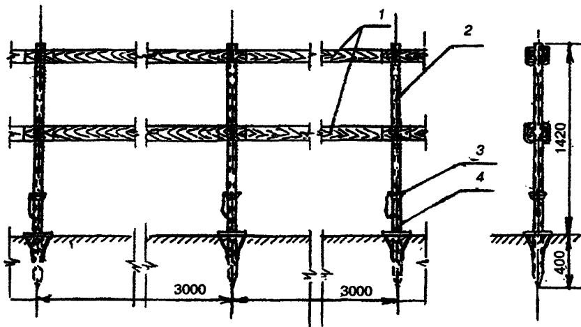
1 — доска; 2 — стойка; 3 — стопор; 4 — основание
