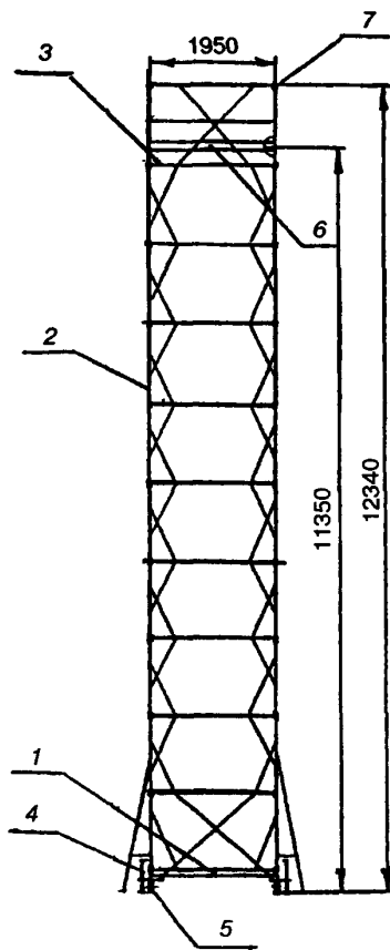
1 — база; 2 — лестница; 3 — стяжки; 4 — винтовая опора; 5 — колесный блок; 6 — настил; 7 — поручень
