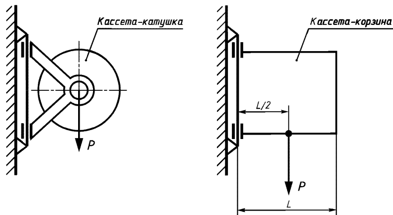
Рисунок 1 — Схема приложения нагрузки P к поворотной кассете
