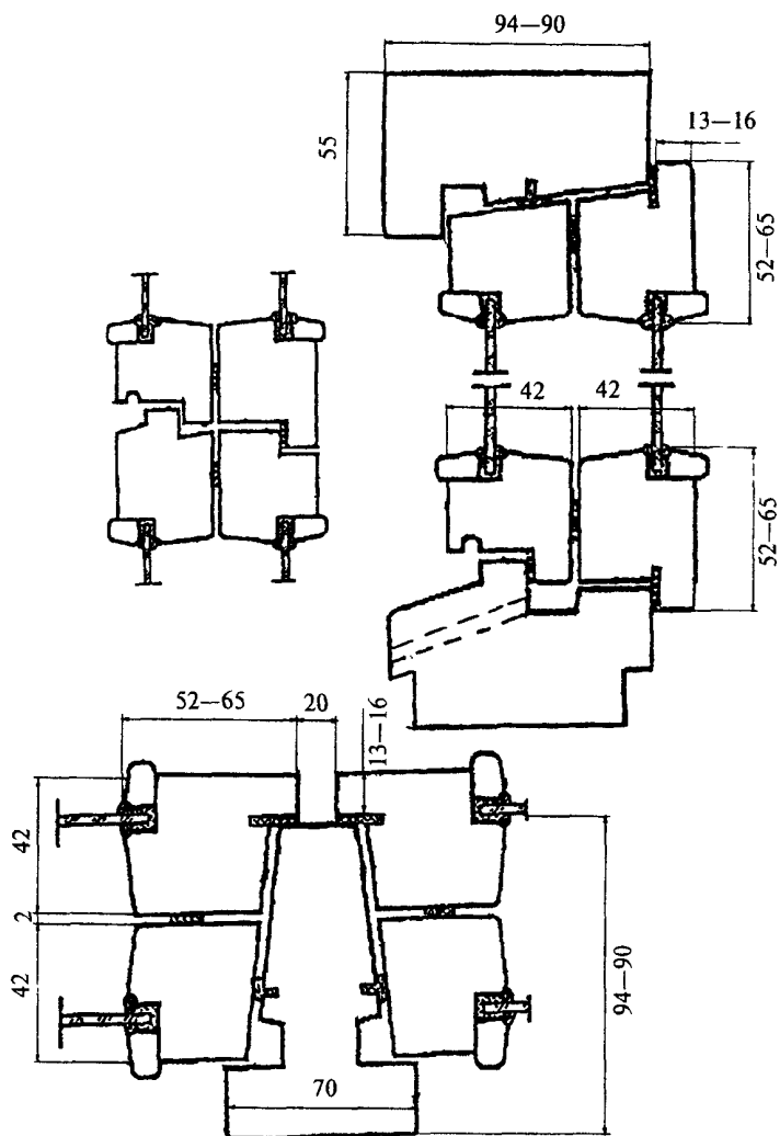
Рисунок 3 – Примеры конструктивных решений оконных блоков спаренной конструкции (с распашным открыванием створок, двумя рядами уплотняющих прокладок, наплав толщиной 16 мм – под ввертную петлю)
