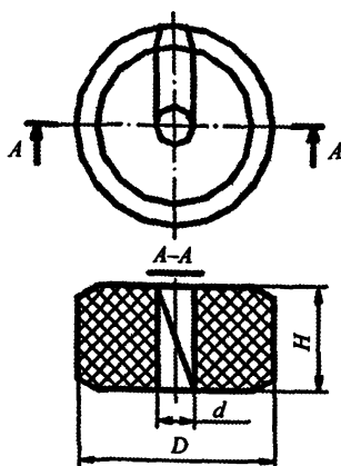
Рис. П6.2. Кольцо для уплотнения кабелей
