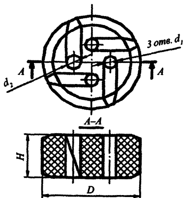
Рис. П6.1. Кольцо для уплотнения проводов
