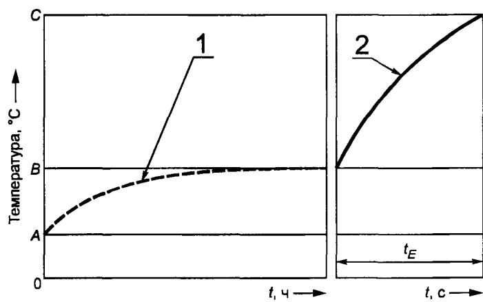
А — наивысшая допустимая окружающая температура; В — температура в номинальном режиме работы; С — предельная температура; t — время; 1 — повышение температуры в номинальном режиме работы; 2 — повышение температуры статора и ротора при испытании электродвигателя с заторможенным ротором
