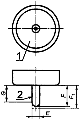
1 — изоляционный материал (вид произвольный); 2 — полированная поверхность для припаивания
