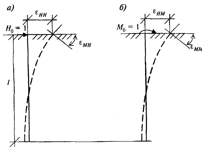
Рисунок Д.2 — Схема перемещений сваи в грунте
