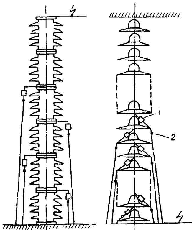
Установка регистраторов перекрытий на испытываемых объектах: 1 - регистратор перекрытий; 2 - грузик
