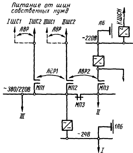
Рис.5. Структурные схемы питания узла СДТУ электростанций
