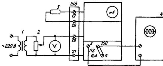
Рис.29. Схема для проверки характеристики манипуляции:
