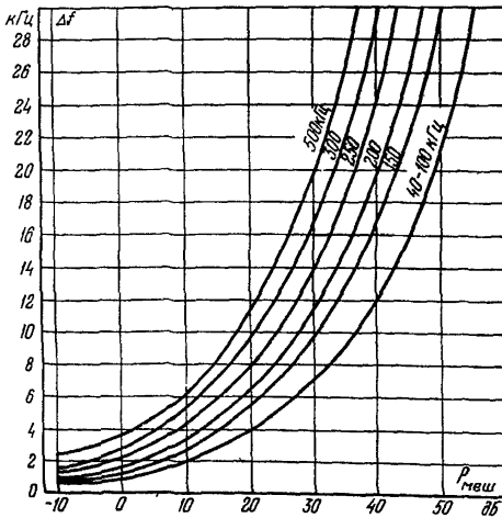
Рис.16. Характеристики допустимых уровней мешающего сигнала для приемника УПЗ-70 при работе без линейного фильтра и при разности частот передачи и приема не менее 10%
