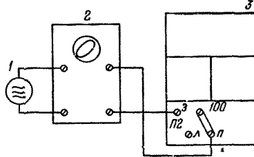
Рис. 22. Схема для проверки частоты передатчика методом сравнения по фигурам Лиссажу: 1 - ВЧ генератор; 2 - осциллограф; 3 - приемопередатчик
