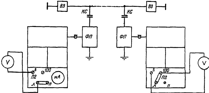
Рис.32. Схема для измерения затухания ВЧ канала
