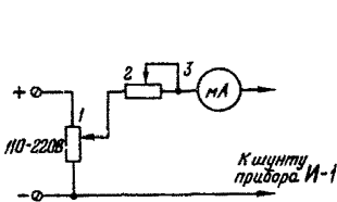
Рис. 21. Схема для проверки прибора И-1:
