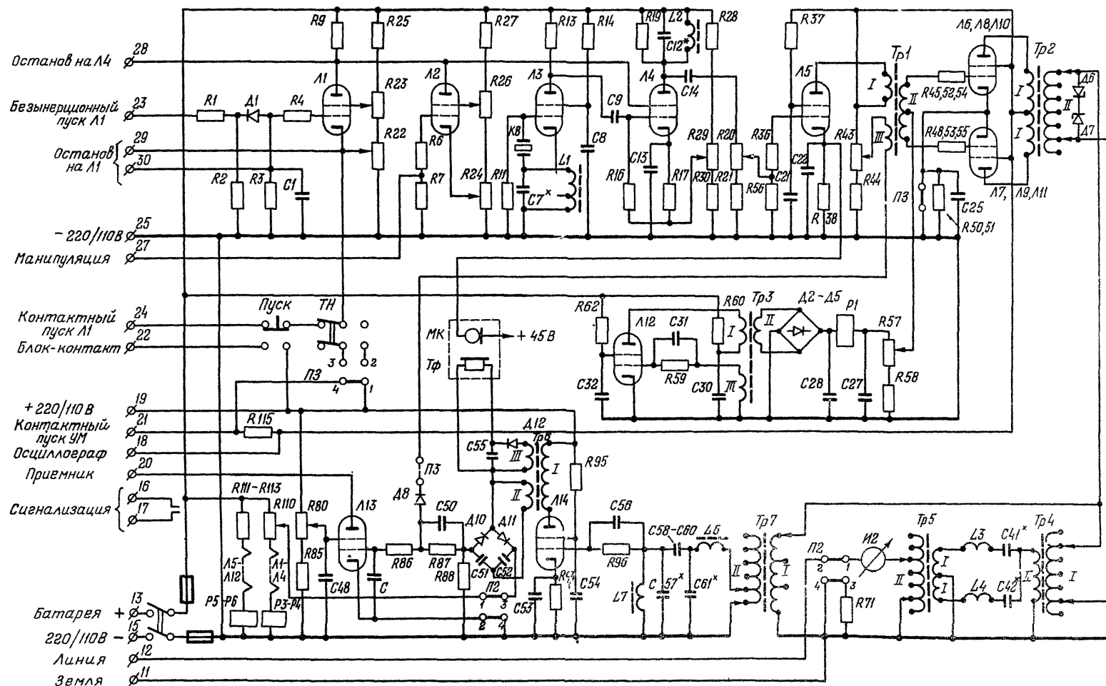
Рис.2. Упрощенная принципиальная схема приемопередатчика УПР-70
