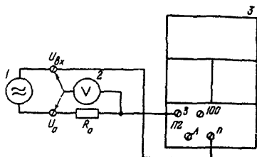
Рис.25. Схема для измерения входного сопротивления приемопередатчика: R_0 = 10 \div 50 \text{ Ом} Обозначения см. на рис. 23.
