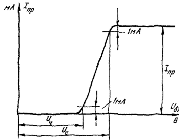
Рис.13. Характеристика чувствительности приемника при работе с направленной антенной
