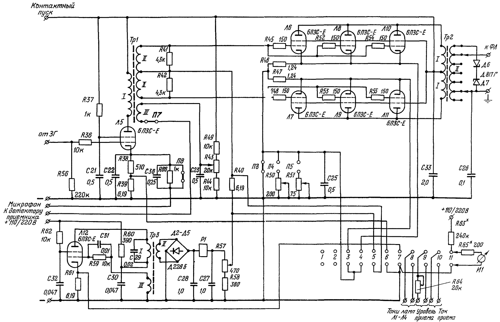
Рис.5. Схема усилителя мощности и генератора смещения
