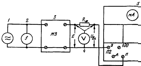
Рис.28. Схема для проверки характеристики избирательности приемника при работе передатчика с дифференциально-мостиковым ФЛ:
