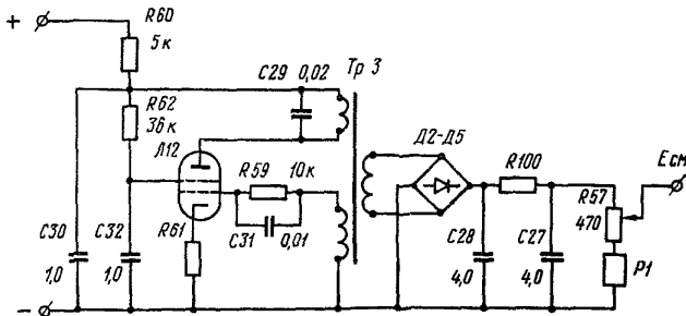
Рис.37. Принципиальная схема генератора смещения (измененная)
