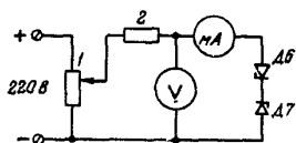
Рис.26. Схема для определения напряжения срабатывания стабилизаторов Д6, Д7:
