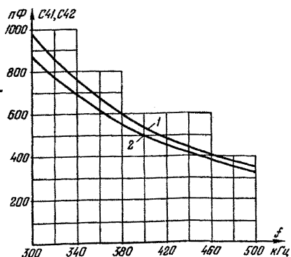
Рис.40. Зависимость значения емкости контуров ФЛ от заданной частоты настройки (диапазон частот 301-500 кГц; L3 = L4 = 0,3 мГ):
