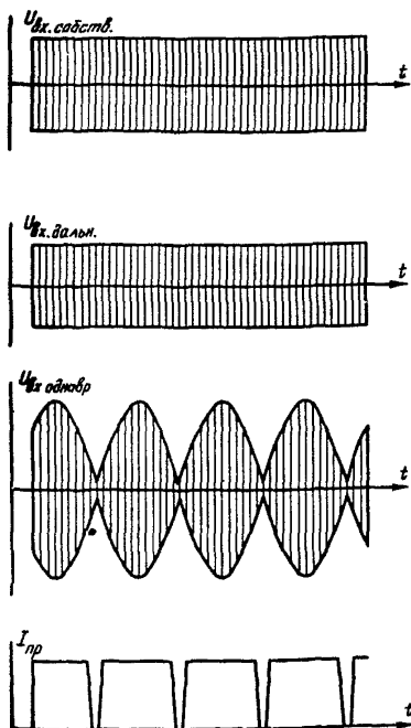
Рис. 20. Биения на входе приемника для случая, когда амплитуда напряжения на входе приемника при пуске собственного передатчика близка к амплитуде напряжения, принимаемого от дальнего передатчика
