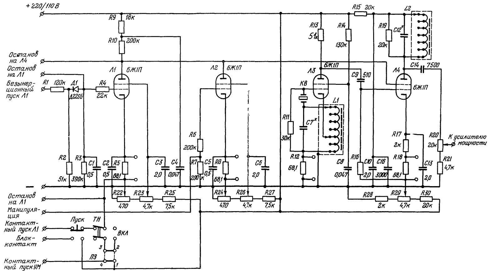
Рис.3. Схема блока управления и задающего генератора (перемычки показаны для работы с защитой ДФБ-500)
