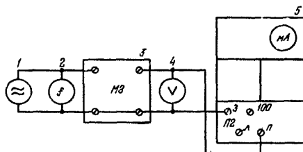
Рис.27. Схема для настройки приемника и для проверки характеристики чувствительности:
