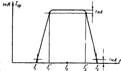
Рис.17. Характеристика избирательности приемника при работе с направленной защитой
