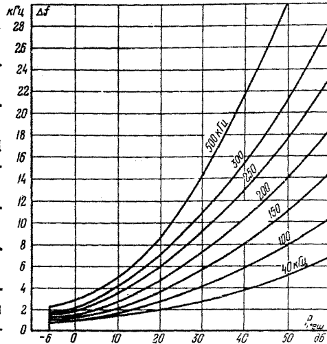
Рис.15. Характеристики допустимых уровней мешающего сигнала для приемника УПС-70 при работе с линейным фильтром на одной частоте или с разнесом частот до 2 кГц
