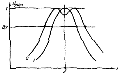
Рис.12. Частотная характеристика приемного фильтра:
