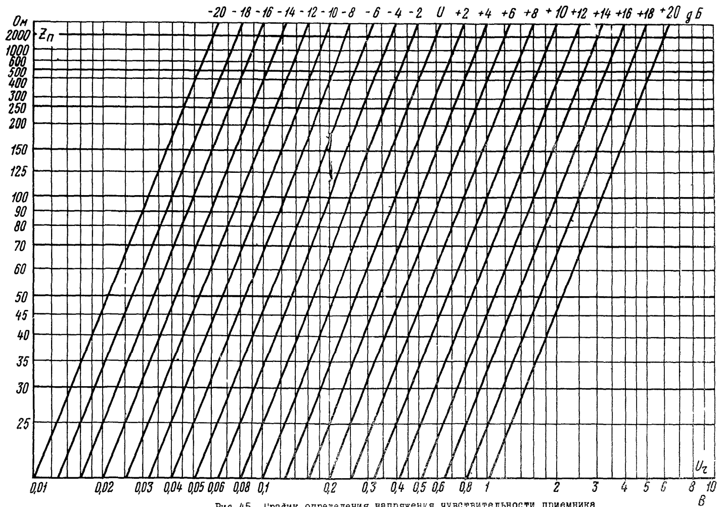
Рис.45. График определения напряжения чувствительности приемника при заданном уровне чувствительности (для Z_n = 100 \text{ Ом} )
