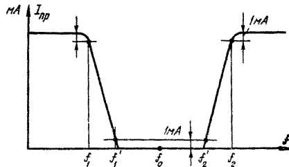
Рис.18. Характеристика избирательности приемника при работе с дифференциально-фазной защитой
