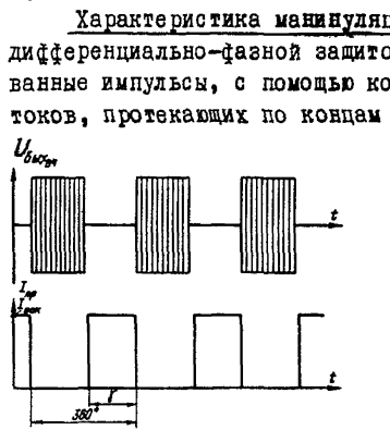
Рис. 9. Форма манипулируемых ВЧ сигналов на выходе передатчика и соответствующие им импульсы тока приемника
