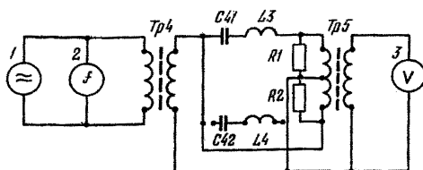
Рис.41. Схема для настройки контура ФЛ:
