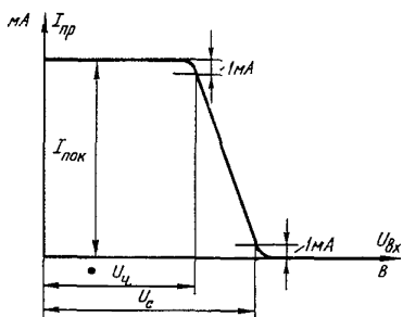
Рис.14. Характеристика чувствительности приемника при работе с дифференциально-фазной защитой
