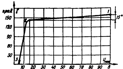
Рис. 10. Характеристика манипуляции: 1 - точка, соответствующая максимальной ширине импульса тока приемника; 2 - точка, соответствующая напряжению полной манипуляции; 3 - начало действия манипулятора
