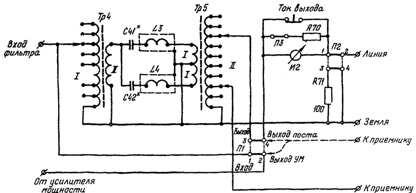
Рис.6. Схема линейного фильтра
