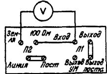
Рис.32. Схема для измерения затухания ВЧ канала
