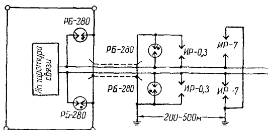
Рис.7. Защита разрядниками кабельных вводов
